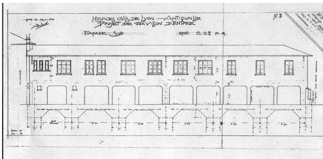
Projet de pavillon d'entrée [23]. N° 5. Façade sud, par Delaval, 1931
