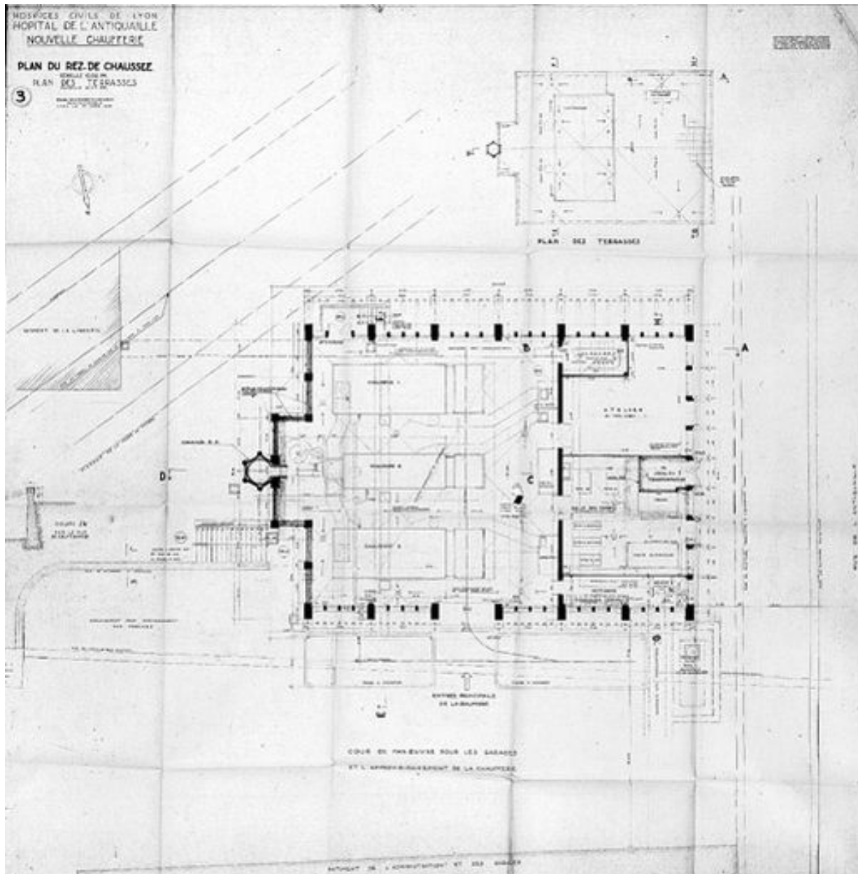
Nouvelle chaufferie. 3. Plan du rez-de-chaussée. Plan des terrasses, par Pierre Bourdeix et Louis Weckerlin, 1955
