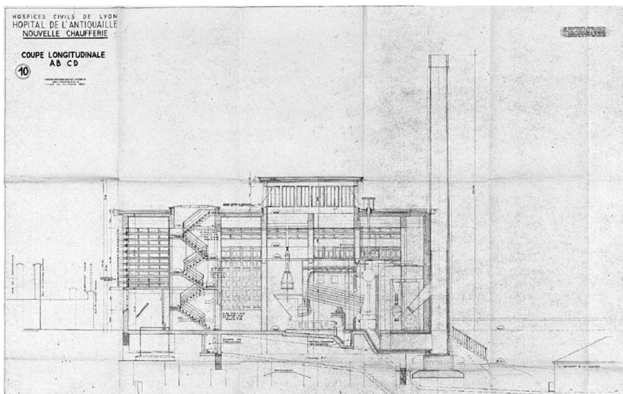
Nouvelle chaufferie. 10. Coupe longitudinale AB CD, par Pierre Boudeix et Louis Weckerlin, 1955
