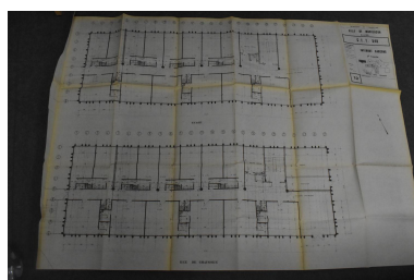
Plan du bâtiment d'internat des garçons, rez-de-chaussée et étage, par le cabinet Lagneau, 25 octobre 1976 (AC Montluçon. 4 M 53/7). Repro. Bénédicte Renaud-Morand, Autr. Paul Lagneau
