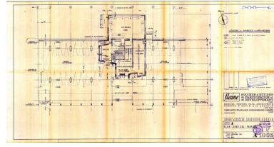
Hôtel A. Plan du sous-sol, parking. Marcel Breuer architecte, Robert F. Gatje associé, 7 novembre 1961. Révision générale 12 décembre 1961 (AC Arâches-la-Frasse) Phot. Jean-François Lyon-Caen, Phot. C. Salomon-Pelen, Autr. Breuer Marcel (architecte), Autr. Gatje Robert F. (architecte) IVR82_20117402071NUC
