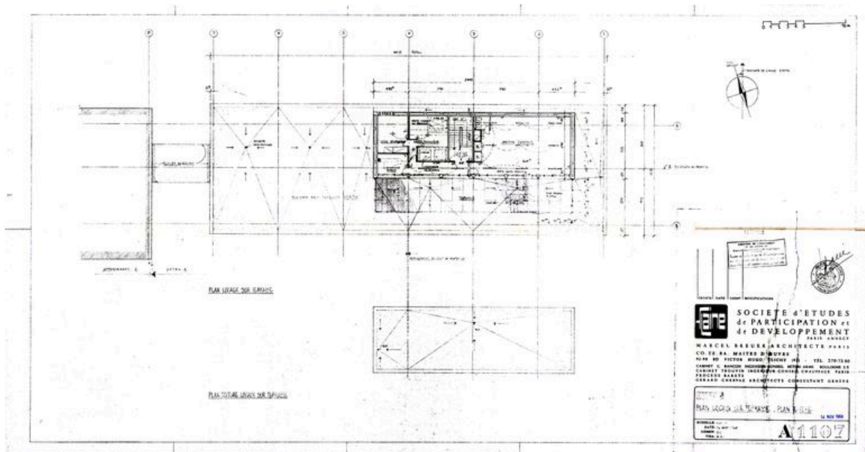
Hôtel A. Plan des locaux sur le toit terrasse. Plan de toiture. Marcel Breuer architecte, 26 août 1968 (AC Arâches-la-Frasse)
