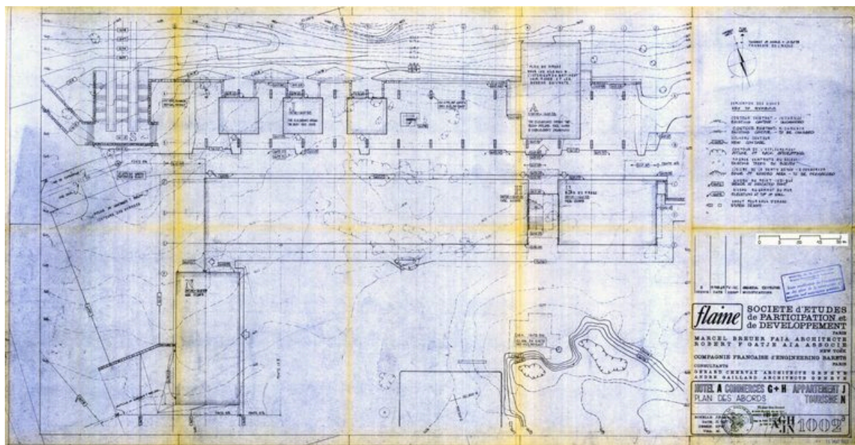
Hôtel A. Commerce G et H. Appartement J. Tourisme N. Plan des abords. Marcel Breuer FAIA architecte, Robert F. Gatje AIA associé, 12 septembre 1962 (AC Arâches-la-Frasse)
