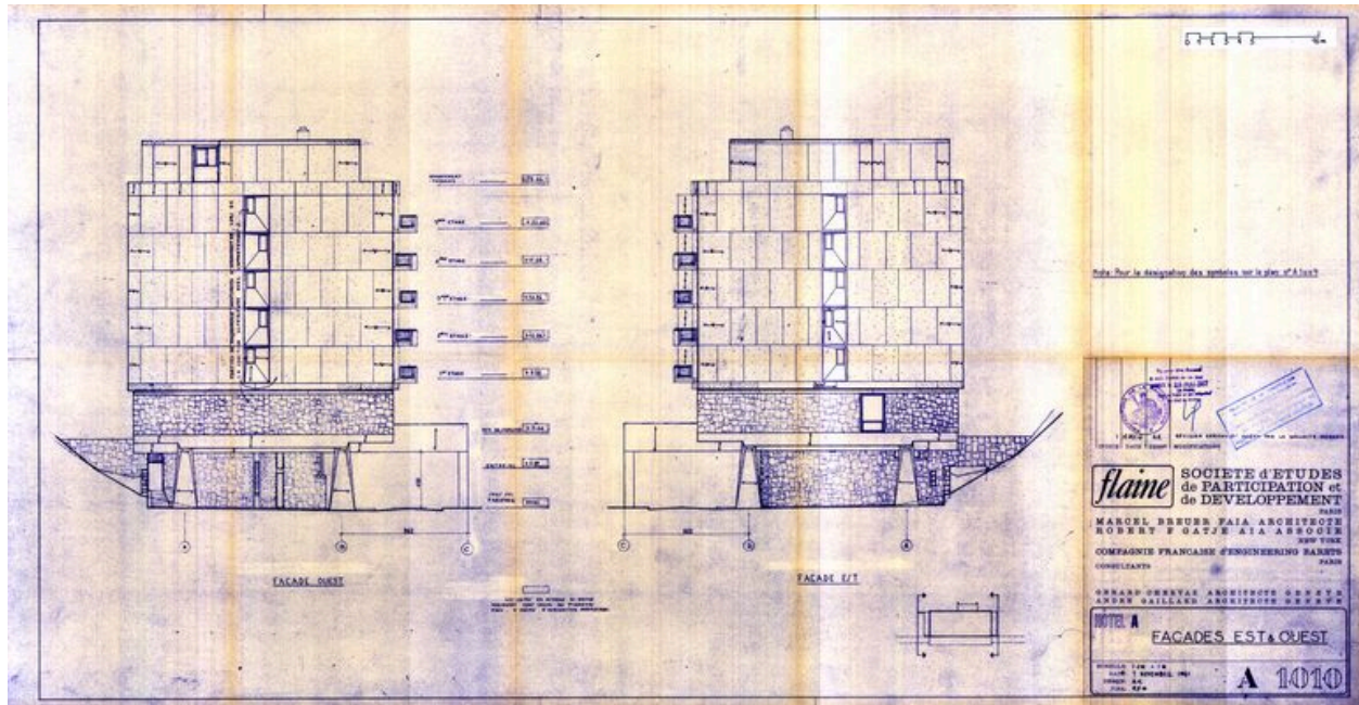
Hôtel A. Elévations est et ouest. Marcel Breuer architecte, Robert F. Gatje associé, 7 novembre 1961. Révision générale 12 décembre 1961 (AC Arâches-la-Frasse)
