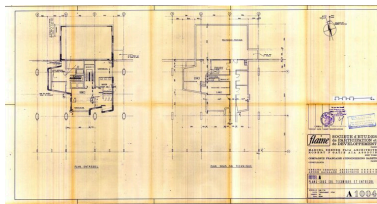
Hôtel A. Plans du sous-sol technique et de l'entresol. Marcel Breuer architecte, Robert F. Gatje associé, 7 novembre 1961. Révision générale 12 décembre 1961 (AC Arâches-la-Frasse) Phot. Jean-François Lyon-Caen, Phot. C. Salomon-Pelen, Autr. Breuer Marcel (architecte), Autr. Gatje Robert F. (architecte) IVR82_20117402073NUC
