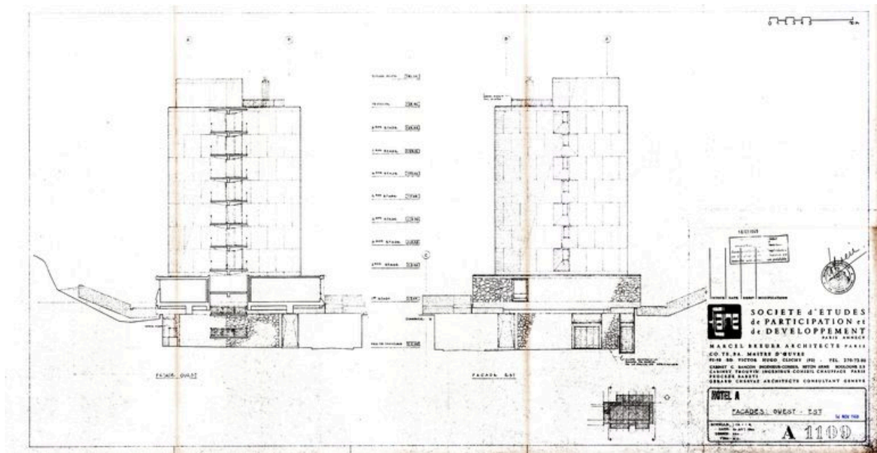
Hôtel A. Elévations ouest et est. Marcel Breuer architecte, 26 août 1968 (AC Arâches-la-Frasse)
