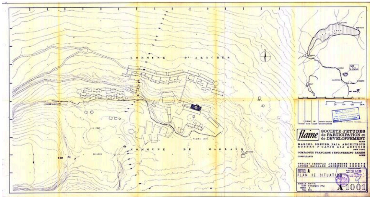
Hôtel A. Plan de situation. Marcel Breuer architecte, Robert F. Gatje associé, 7 novembre 1961. Révision générale 12 décembre 1961 (AC Arâches-la-Frasse)
