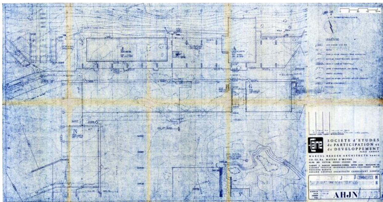
Plan des abords. Marcel Breuer architecte, 10 septembre 1966. Modifications 12 avril et 5 décembre 1967 (AC Arâches-la-Frasse)
