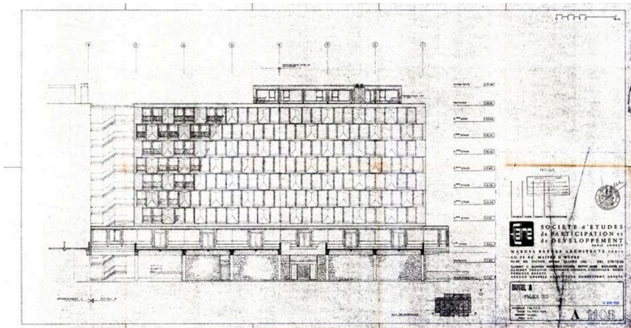
Hôtel A. Elévation sud. Marcel Breuer architecte, 26 août 1968 (AC Arâches-la-Frasse)
