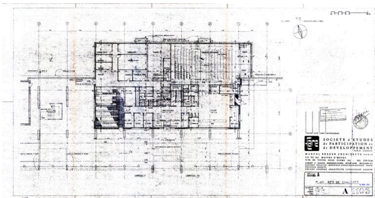
Hôtel A. Plan du rez-de-chaussée. Marcel Breuer architecte, 26 août 1968 (AC Arâches-la-Frasse)
