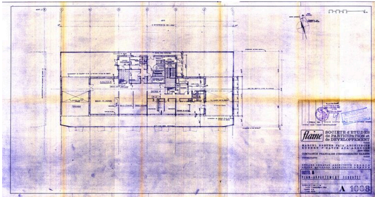
Hôtel A. Plan de l'appartement en terrasse. Marcel Breuer architecte, Robert F. Gatje associé, 7 novembre 1961. Révision générale 12 décembre 1961 (AC Arâches-la-Frasse)
