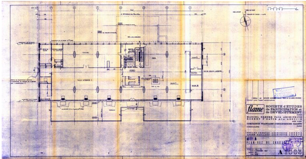
Hôtel A. Plan du rez-de-chaussée. Marcel Breuer architecte, Robert F. Gatje associé, 7 novembre 1961. Révision générale 12 décembre 1961 (AC Arâches-la-Frasse)
