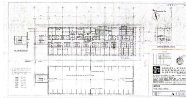
Hôtel A. Plan d'un étage courant. Marcel Breuer architecte, 26 août 1968 (AC Arâches-la-Frasse) Phot. Jean-François Lyon- Caen, Phot. C. Salomon-Pelen, Autr. Breuer Marcel (architecte) IVR82_20117402086NUC
