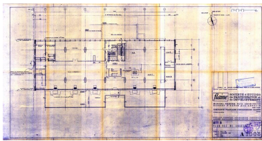
Hôtel A. Plan du rez-de-chaussée. Marcel Breuer architecte, Robert F. Gatje associé, 7 novembre 1961. Révision générale 12 décembre 1961 (AC Arâches-la-Frasse) Phot. Jean-François Lyon-Caen, Phot. C. Salomon-Pelen, Autr. Breuer Marcel (architecte), Autr. Gatje Robert F. (architecte) IVR82_20117402072NUC
