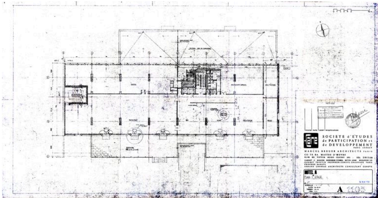
Hôtel A. Plan du 1er étage. Marcel Breuer architecte, 26 août 1968 (AC Arâches-la-Frasse)
