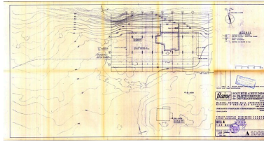
Hôtel A. Plan masse. Marcel Breuer architecte, Robert F. Gatje associé, 7 novembre 1961. Révision générale 12 décembre 1961 (AC Arâches-la-Frasse) Phot. Jean-François Lyon-Caen, Phot. C. Salomon-Pelen, Autr. Breuer Marcel (architecte), Autr. Gatje Robert F. (architecte) IVR82_20117402070NUC
