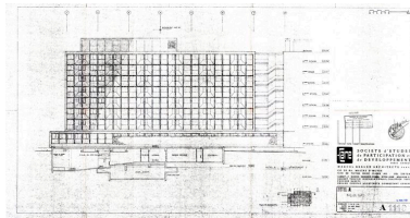
Hôtel A. Elévation nord. Marcel Breuer architecte, 26 août 1968 (AC Arâches-la-Frasse) Phot. Jean-François Lyon- Caen, Phot. C. Salomon-Pelen, Autr. Breuer Marcel (architecte) IVR82_20117402090NUC
