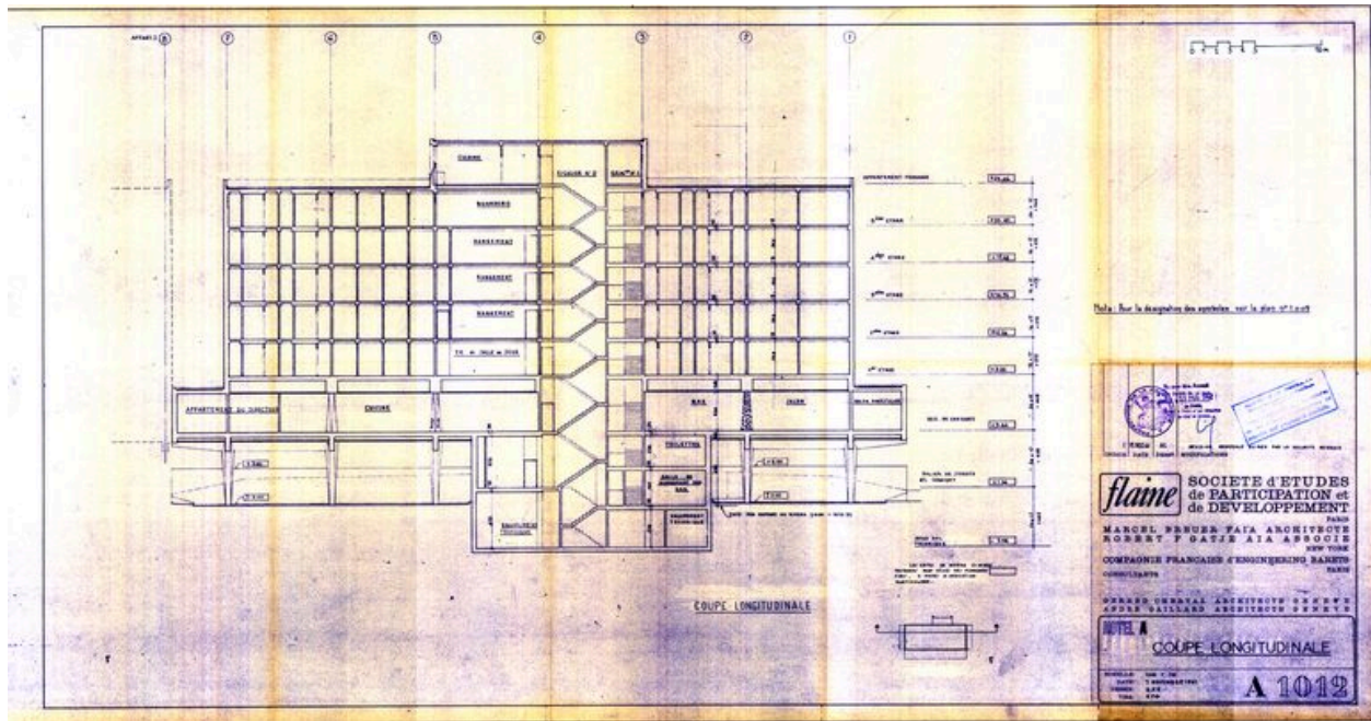
Hôtel A. Coupe longitudinale. Marcel Breuer architecte, Robert F. Gatje associé, 7 novembre 1961. Révision générale 12 décembre 1961 (AC Arâches-la-Frasse)
