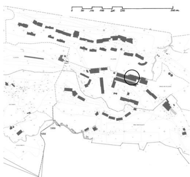
Plan de situation, d'après le plan cadastral d'Arâches-la-Frasse, section CO1, 2006 Dess. Jean-François Lyon-Caen, Dess. C. Salomon-Pelen
