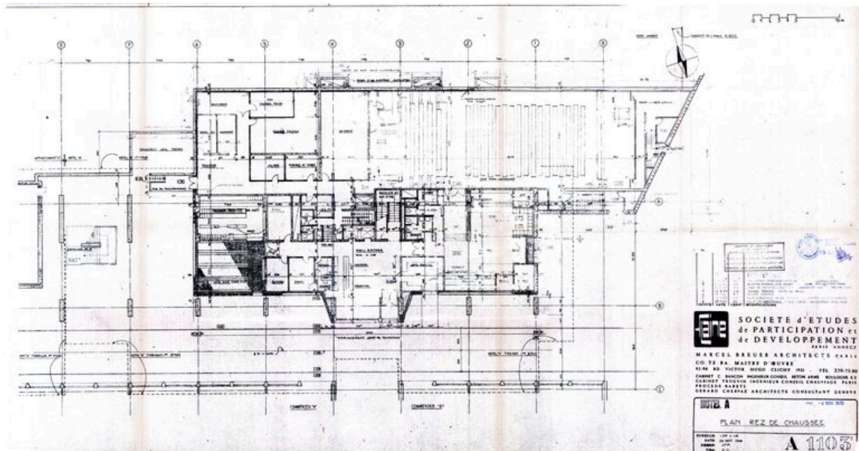
Hôtel A. Plan du rez-de-chaussée. Marcel Breuer architecte, 26 août 1968. Modifié 4 novembre 1970 (AC Arâches-la-Frasse)
