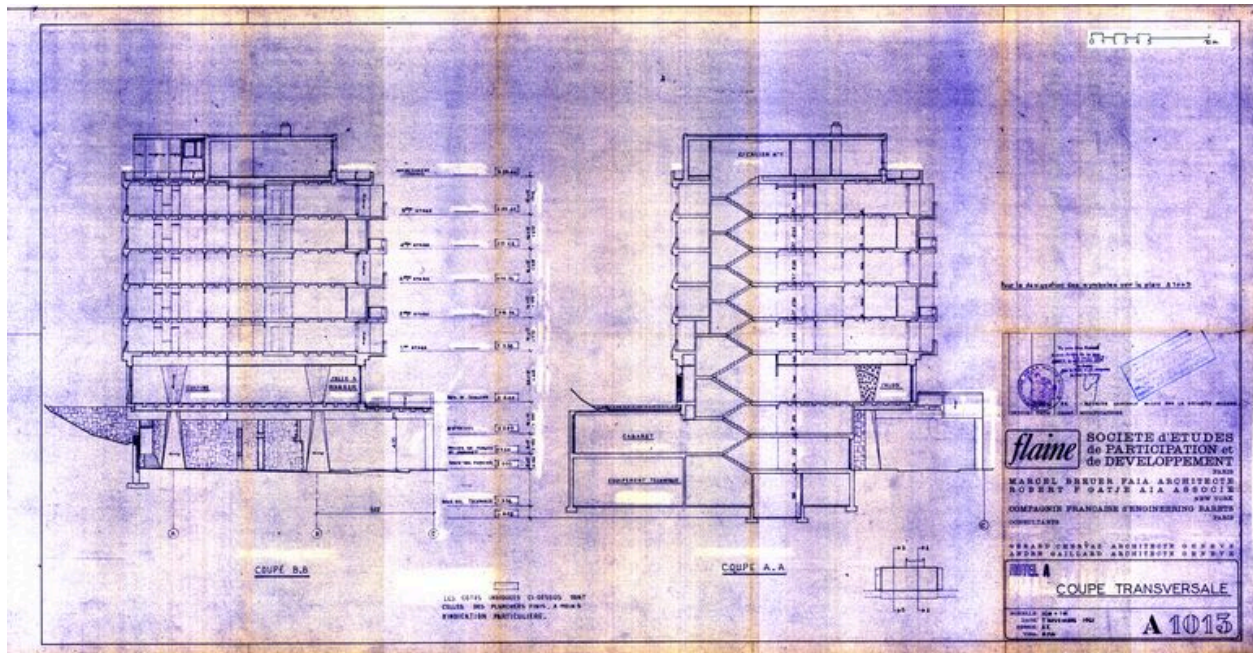
Hôtel A. Coupe transversale. Marcel Breuer architecte, Robert F. Gatje associé, 7 novembre 1961. Révision générale 12 décembre 1961 (AC Arâches-la-Frasse)
