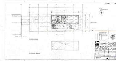
Hôtel A. Plan des locaux sur le toit terrasse. Plan de toiture. Marcel Breuer architecte, 26 août 1968 (AC Arâches-la-Frasse) Phot. Jean-François Lyon- Caen, Phot. C. Salomon-Pelen, Autr. Breuer Marcel (architecte) IVR82_20117402087NUC
