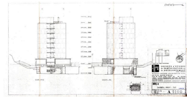
Hôtel A. Elévations ouest et est. Marcel Breuer architecte, 26 août 1968 (AC Arâches-la-Frasse) Phot. Jean-François Lyon- Caen, Phot. C. Salomon-Pelen, Autr. Breuer Marcel (architecte) IVR82_20117402091NUC
