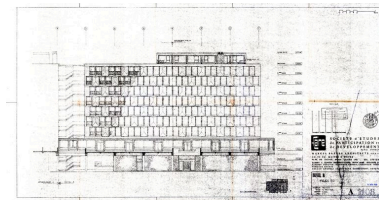
Hôtel A. Elévation sud. Marcel Breuer architecte, 26 août 1968 (AC Arâches-la-Frasse) Phot. Jean-François Lyon- Caen, Phot. C. Salomon-Pelen, Autr. Breuer Marcel (architecte) IVR82_20117402089NUC
