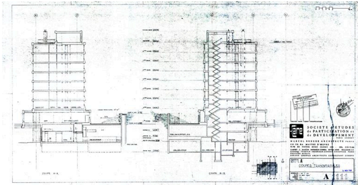
Hôtel A. Coupes transversales. Marcel Breuer architecte, 26 août 1968 (AC Arâches-la-Frasse)
