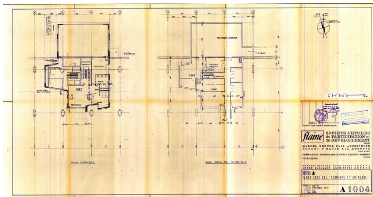
Hôtel A. Plans du sous-sol technique et de l'entresol. Marcel Breuer architecte, Robert F. Gatje associé, 7 novembre 1961. Révision générale 12 décembre 1961 (AC Arâches-la-Frasse)
