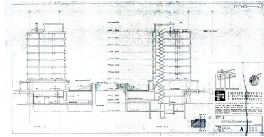
Hôtel A. Coupes transversales. Marcel Breuer architecte, 26 août 1968 (AC Arâches-la-Frasse) Phot. Jean-François Lyon- Caen, Phot. C. Salomon-Pelen, Autr. Breuer Marcel (architecte) IVR82_20117402088NUC
