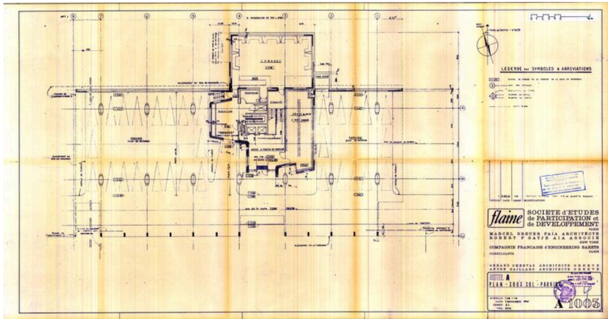
Hôtel A. Plan du sous-sol, parking. Marcel Breuer architecte, Robert F. Gatje associé, 7 novembre 1961. Révision générale 12 décembre 1961 (AC Arâches-la-Frasse)
