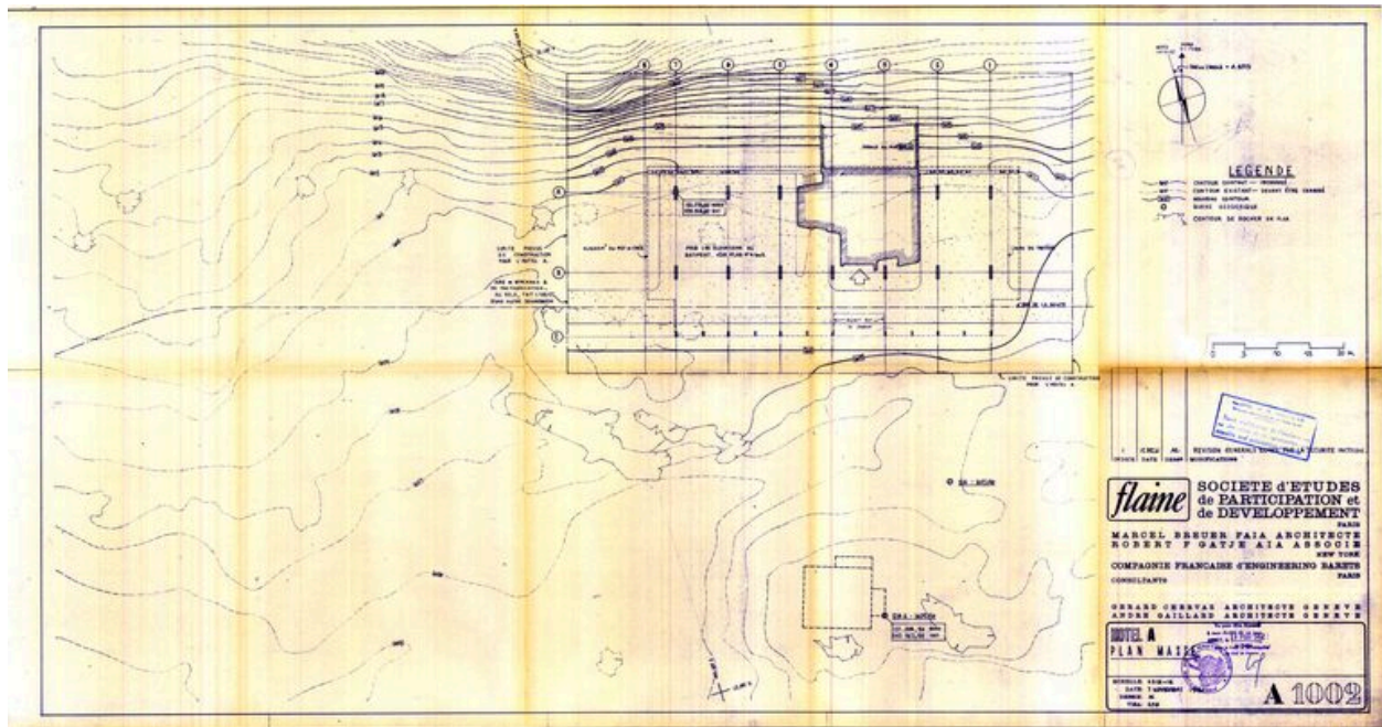
Hôtel A. Plan masse. Marcel Breuer architecte, Robert F. Gatje associé, 7 novembre 1961. Révision générale 12 décembre 1961 (AC Arâches-la-Frasse)
