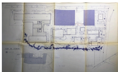
Plan masse et de situation du CET avec emplacement de la décoration prévue par Albert Féraud (AN, 19880466/116) Repro. Catherine Guégan, Autr. Pierre Adolphe Le Breton IVR84_20236300093NUCA
