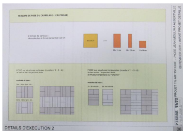
Principes de pose du carrelage. Autr. Pierre Tatu, Autr. Valérie Pamart IVR84_20207300713NUCAB
