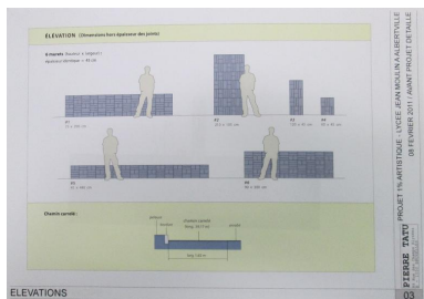
Élévations, avec cotations. Autr. Pierre Tatu, Repro. Valérie Pamart IVR84_20207300712NUCAB
