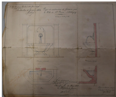
Projet de construction de fontaine pour la ville de Saint-Pierre- d'Albigny. Élévation principale. Élévation latérale. Plan. Coupe / Joseph Samuel Revel (architecte), 21 janvier 1862 (AD Savoie. 20 2691). Phot. Caroline Guibaud, Phot. Joseph-Samuel Revel IVR84_20257300629NUCA
