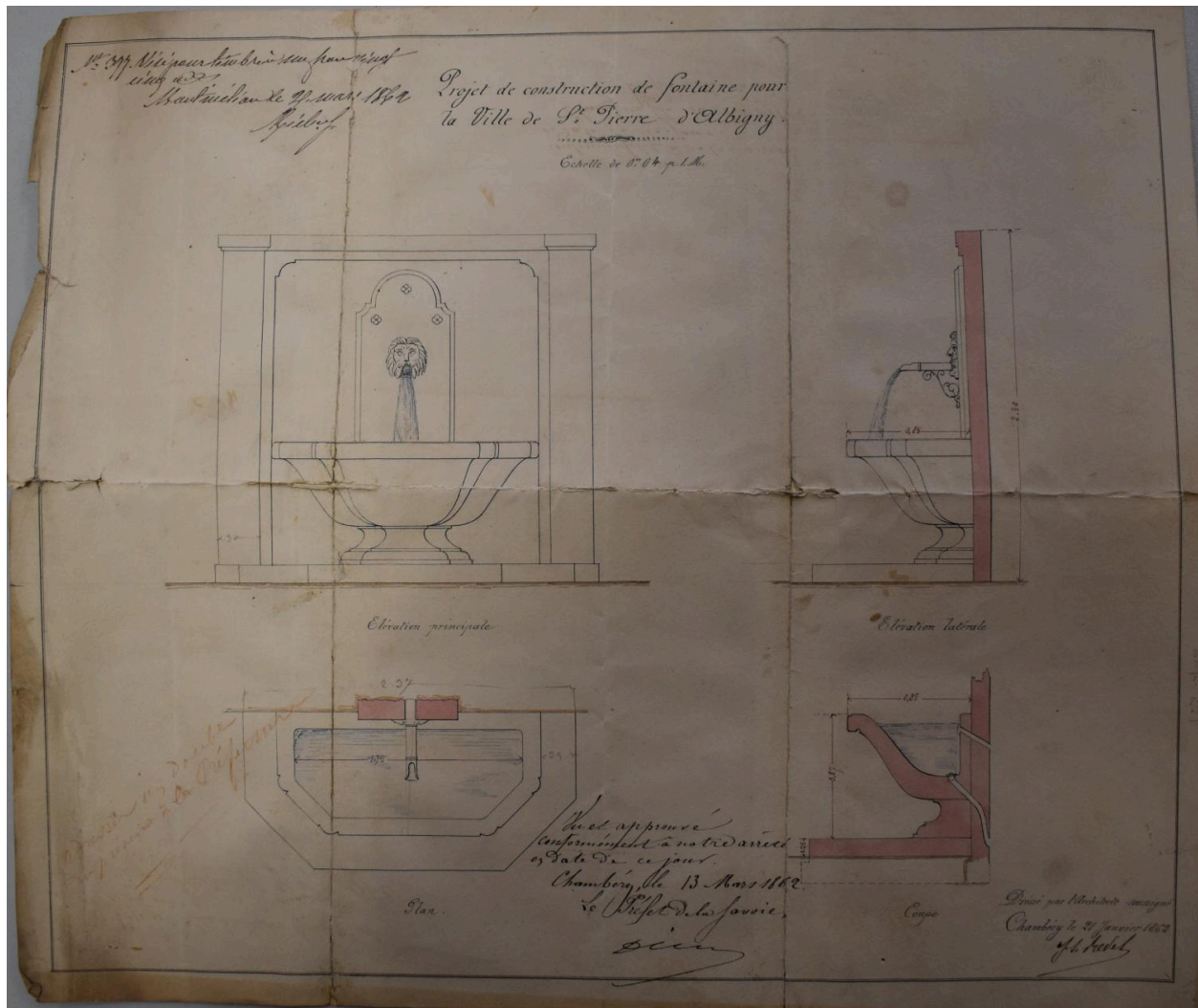
Projet de construction de fontaine pour la ville de Saint-Pierre-d'Albigny. Elévation principale. Elévation latérale. Plan. Coupe / Joseph Samuel Revel (architecte), 21 janvier 1862 (AD Savoie. 2O 2691).
