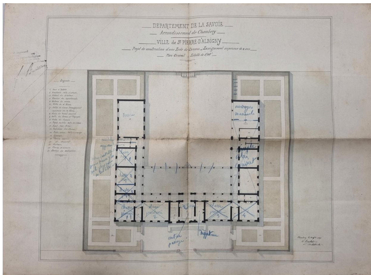
Ville de Saint-Pierre-d'Albigny. Projet de construction d'une école de garçons. Enseignement supérieur de 2 ans [1] Plan général. Echelle de 0,005. Charles Coustard (architecte), 1881 (AD Savoie. 2O 2695).
