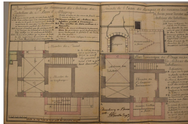
Plan géométrique du bâtiment des archives du tabellion de Saint-Pierre-d'Albigny... 1758, F. A. Garella ingénieur (AD Savoie. 138Edépôt 30). Phot. Caroline Guibaud, Autr. François Antoine Garella IVR84_20257300625NUCA
