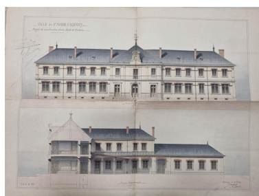
Ville de Saint-Pierre-d'Albigny. Projet de construction d'une école de garçons. Enseignement supérieur de 2 ans [3] Façade principale. Coupe transversale. Echelle de 0,01. Charles Coustard (architecte), 1881 (AD Savoie. 20 2695). Phot. Caroline Guibaud, Autr. Charles Coustard IVR84_20257300640NUCA
