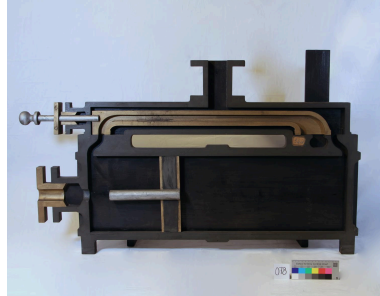
Modèle de piston, vue de face Phot. Krystelle Besson , Phot. Mirco Meier, Phot. Marion Petit IVR84_20256901123NUCA
