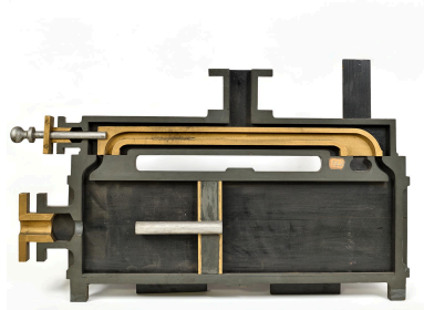
Maquette de piston Phot. Thierry Leroy IVR84_20256901858NUCA
