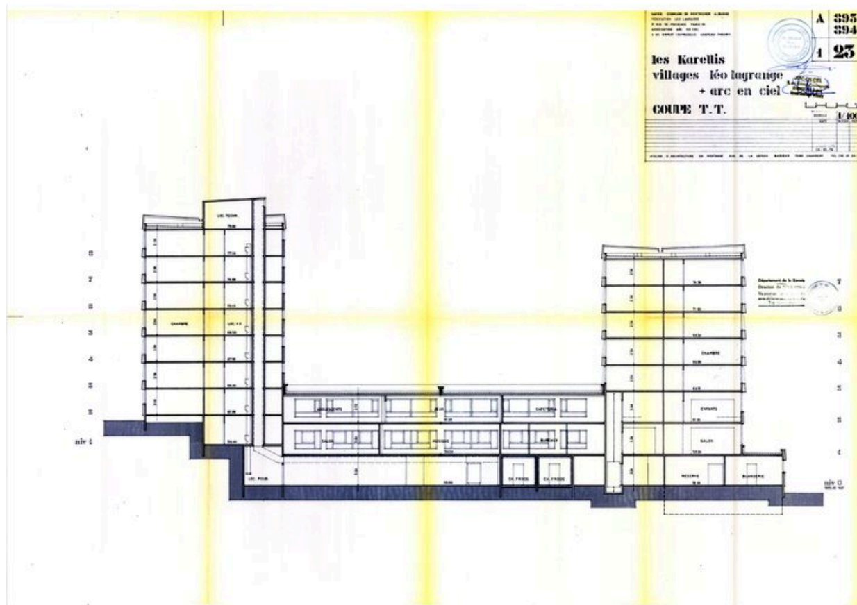
Villages Léo Lagrange et Arc-en-Ciel. Coupe TT (transversale) / Atelier d'architecture en Montagne, Jean Gustav Orth, 20 mai, 5 juin 1976 (AC Montricher-Albanne)
