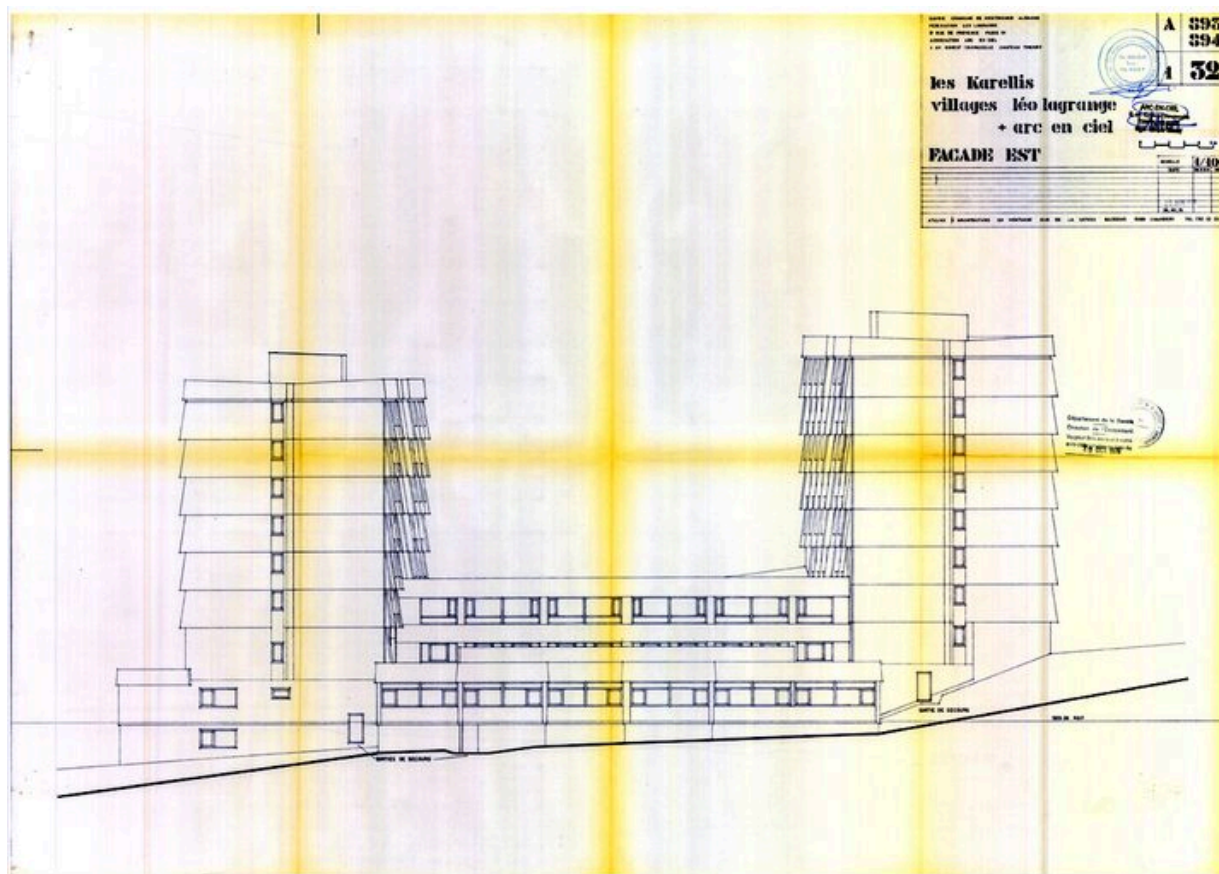
Villages Léo Lagrange et Arc-en-Ciel. Façade est / Atelier d'architecture en Montagne, Jean Gustav Orth, 20 mai, 5 juin 1976 (AC Montricher-Albanne)
