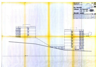
Villages Léo Lagrange et Arc-en-Ciel. Façade ouest / Atelier d'architecture en Montagne, Jean Gustav Orth, 20 mai, 5 juin 1976 (AC Montricher-Albanne) Phot. Jean-François Lyon-Caen IVR82_20127302485NUC
