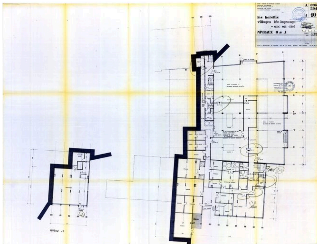
Villages Léo Lagrange et Arc-en-Ciel. Plans niveaux 0 et -1 (accueil) / Atelier d'architecture en Montagne, Jean Gustav Orth, 20 mai, 5 juin 1976 (AC Montricher-Albanne)
