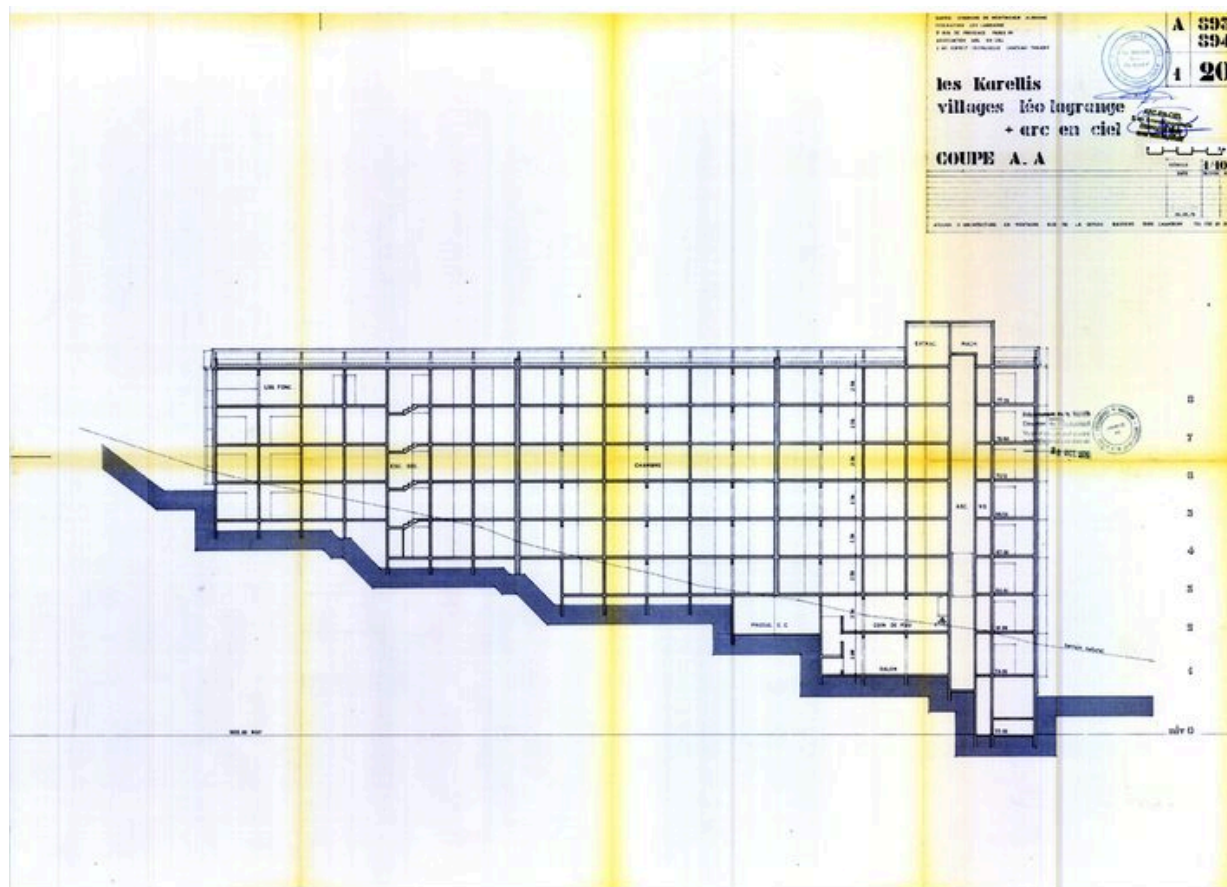
Villages Léo Lagrange et Arc-en-Ciel. Coupe AA (longitudinale sur Balcons de Maurienne) / Atelier d'architecture en Montagne, Jean Gustav Orth, 20 mai, 5 juin 1976 (AC Montricher-Albanne)
