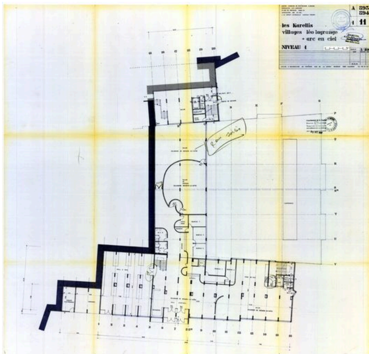
Villages Léo Lagrange et Arc-en-Ciel. Plan niveau 1 / Atelier d'architecture en Montagne, Jean Gustav Orth, 20 mai, 5 juin 1976 (AC Montricher-Albanne)
