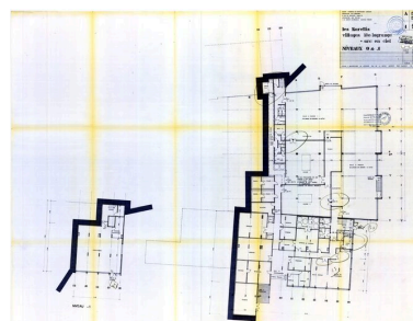
Villages Léo Lagrange et Arc-en-Ciel. Plans niveaux 0 et -1 (accueil) / Atelier d'architecture en Montagne, Jean Gustav Orth, 20 mai, 5 juin 1976 (AC Montricher-Albanne) Phot. Jean-François Lyon-Caen IVR82_20127302472NUC
