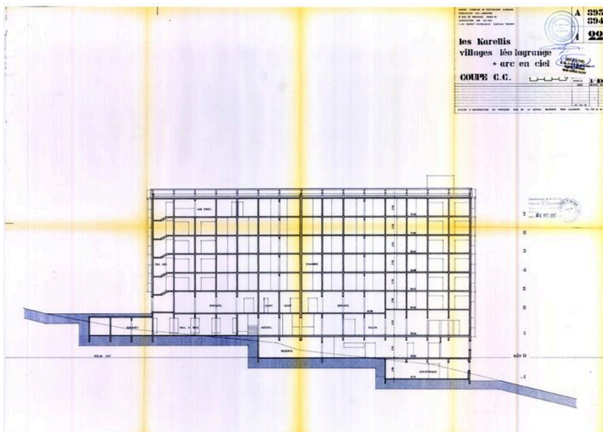
Villages Léo Lagrange et Arc-en-Ciel. Coupe CC (longitudinale sur Arc-en-Ciel) / Atelier d'architecture en Montagne, Jean Gustav Orth, 20 mai, 5 juin 1976 (AC Montricher-Albanne)
