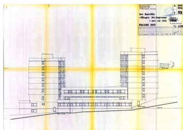
Villages Léo Lagrange et Arc-en-Ciel. Façade est / Atelier d'architecture en Montagne, Jean Gustav Orth, 20 mai, 5 juin 1976 (AC Montricher-Albanne) Phot. Jean-François Lyon-Caen IVR82_20127302486NUC
