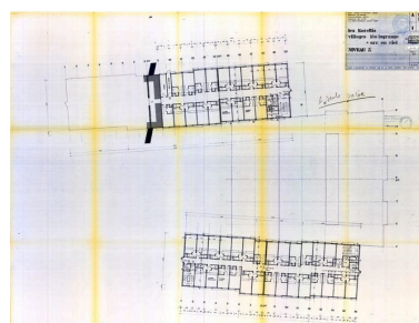
Villages Léo Lagrange et Arc-en-Ciel. Plan niveau 3 (Balcons de Maurienne et Arc-en-Ciel) / Atelier d'architecture en Montagne, Jean Gustav Orth, 20 mai, 5 juin 1976 (AC Montricher-Albanne) Phot. Jean-François Lyon-Caen IVR82_20127302473NUC
