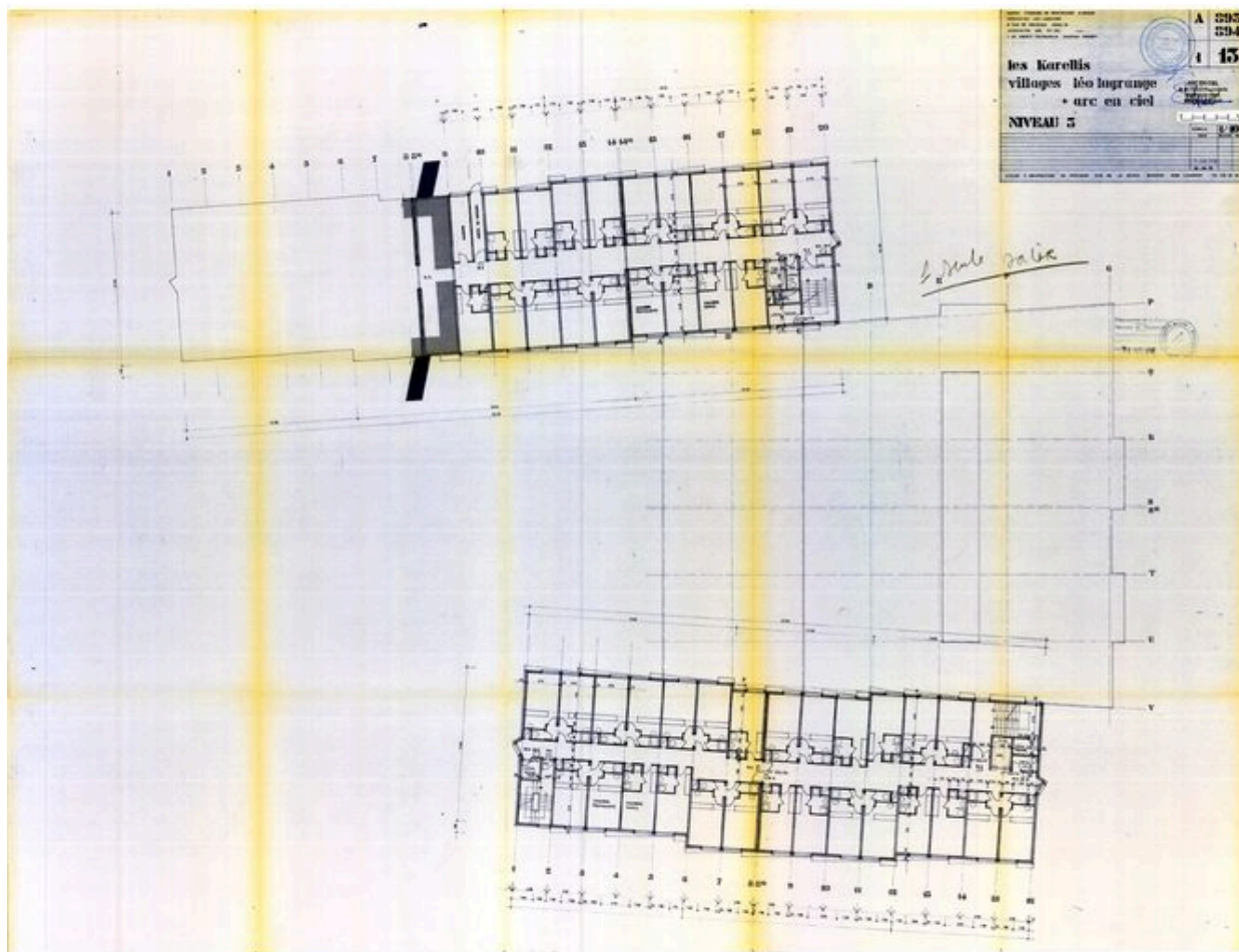
Villages Léo Lagrange et Arc-en-Ciel. Plan niveau 3 (Balcons de Maurienne et Arc-en-Ciel) / Atelier d'architecture en Montagne, Jean Gustav Orth, 20 mai, 5 juin 1976 (AC Montricher-Albanne)
