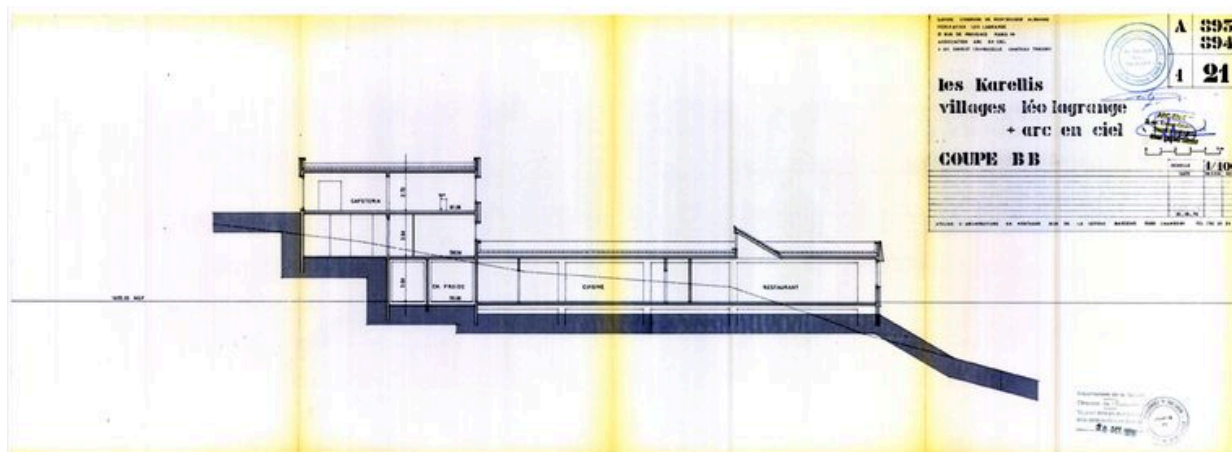
Villages Léo Lagrange et Arc-en-Ciel. Coupe BB (longitudinale sur l'accueil) / Atelier d'architecture en Montagne, Jean Gustav Orth, 20 mai, 5 juin 1976 (AC Montricher-Albanne)
