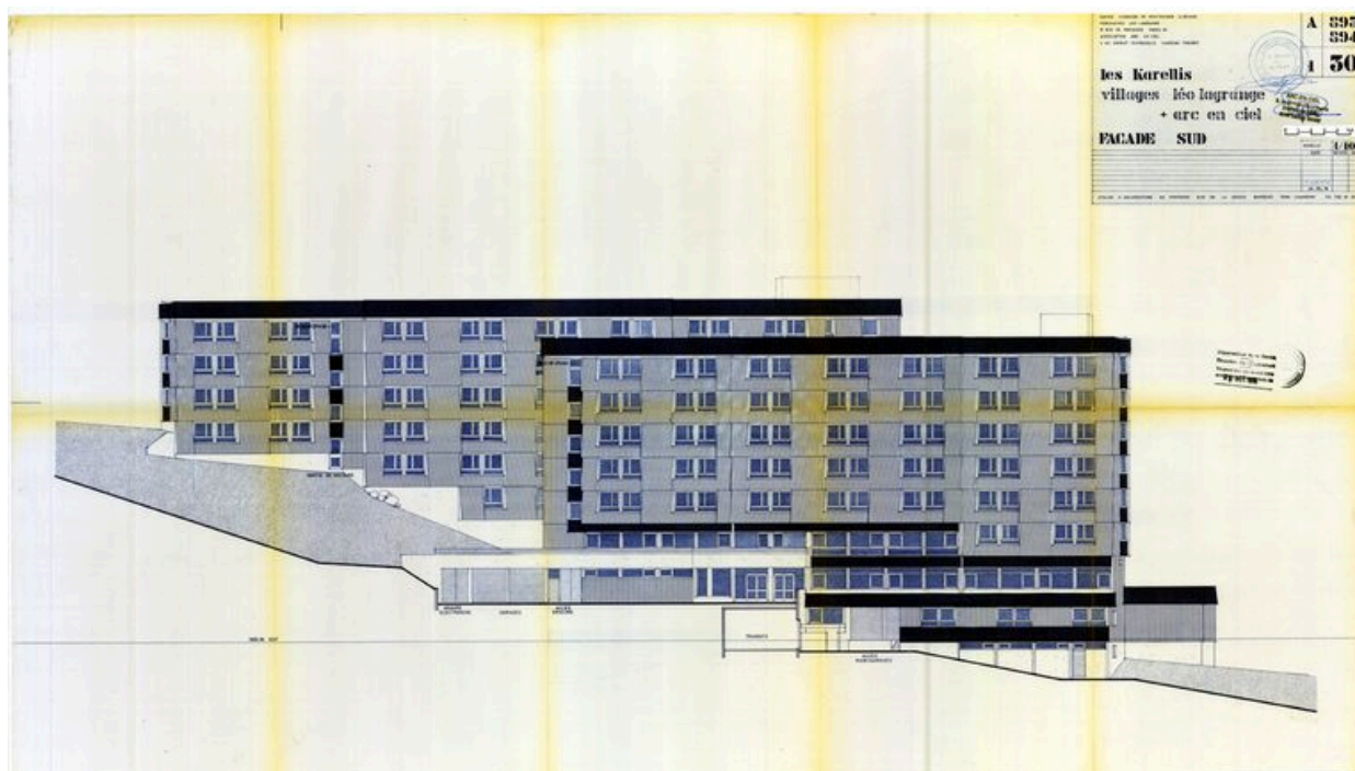
Villages Léo Lagrange et Arc-en-Ciel. Façade sud / Atelier d'architecture en Montagne, Jean Gustav Orth, 20 mai, 5 juin 1976 (AC Montricher-Albanne)
