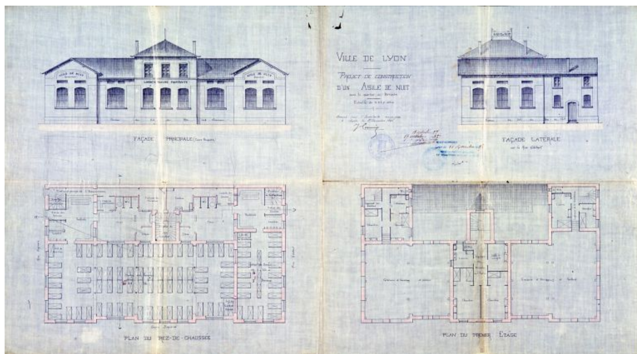
Plans et élévations de l'asile de nuit / J. Cumin, 1886 (AM Lyon)
