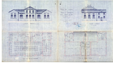
Plans et élévations de l'asile de nuit / J. Cumin, 1886 (AM Lyon) Phot. Jacques Gastineau, Autr. Cumin J. (architecte) IVR82_20026903942NUCA
