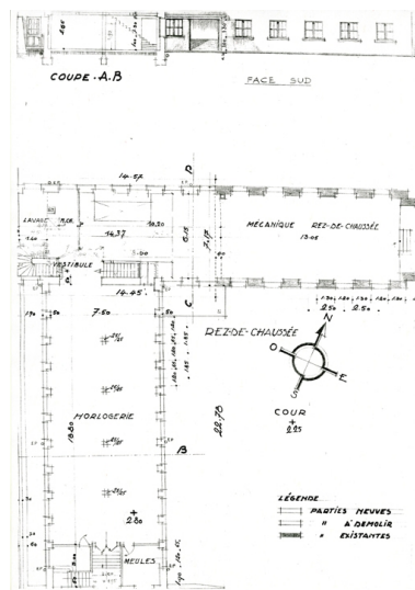
Plan masse rez-de-chaussée Phot. Nadine Halitim-Dubois IVR82_20057400020NUC
