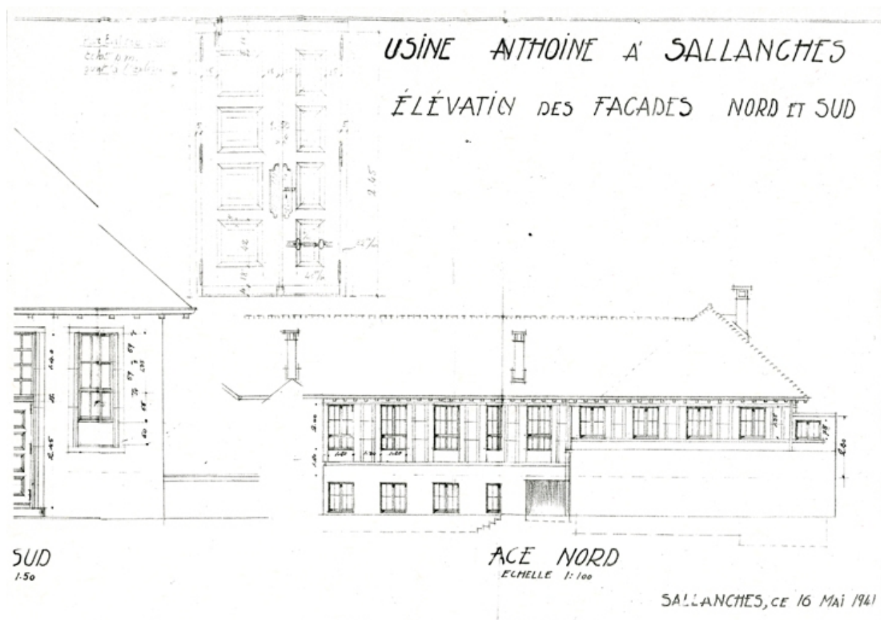
Elévation façade nord (S. Weber architecte) 1941
