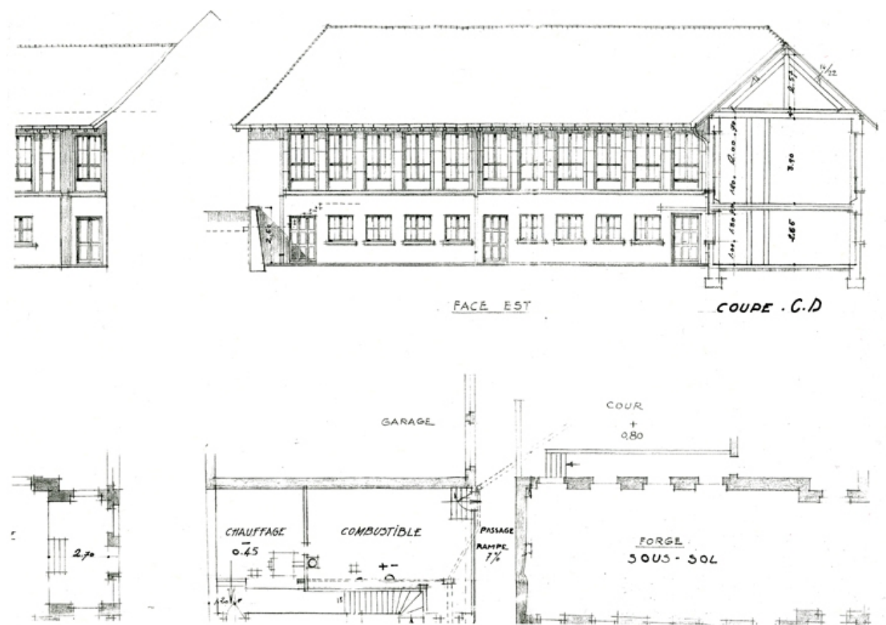
Coupe façade est
