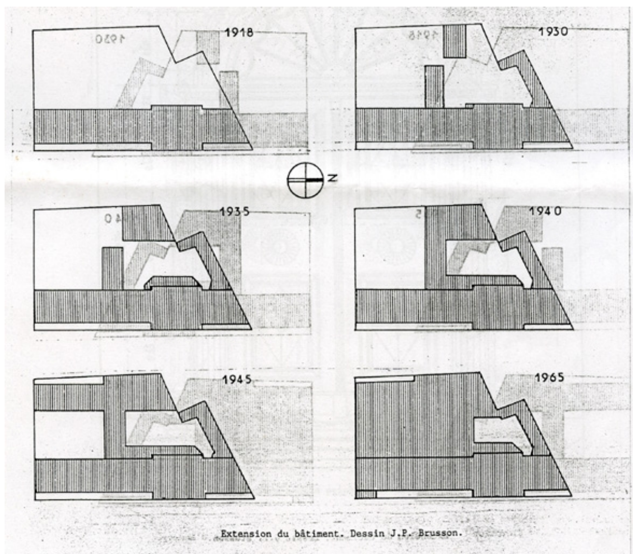
Extension du bâtiment, dessin J-P. Brusson architecte
