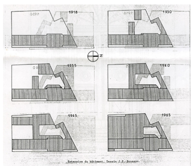
Extension du bâtiment, dessin J-P. Brusson architecte Phot. Nadine Halitim-Dubois IVR82_20077400059NUC
