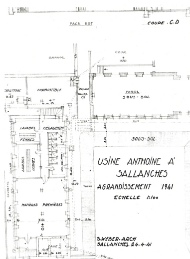
Plan masse 1941 : agrandissement de l'usine Anthoine Phot. Nadine Halitim-Dubois IVR82_20057400021NUC
