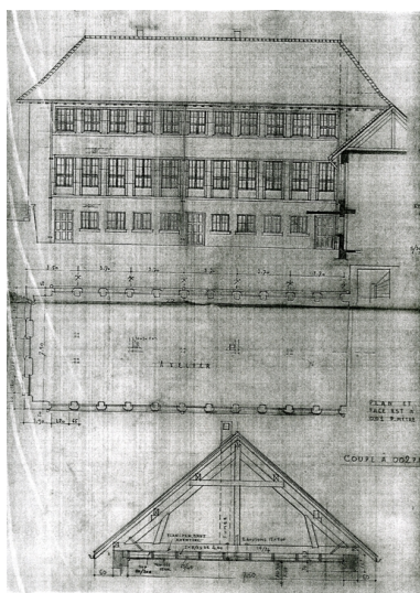
Plan et façade est Phot. Nadine Halitim-Dubois IVR82_20057400018NUC
