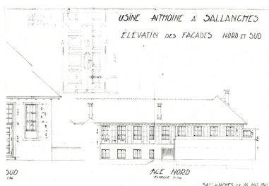
Elévation façade nord (S. Weber architecte) 1941 Phot. Nadine Halitim-Dubois IVR82_20057400015NUC
