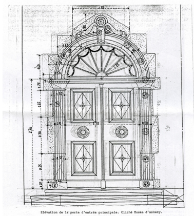
Elévation de la porte d'entrée principale. Cliché Musée d'Annecy (Brusson J-Paul) Phot. Nadine Halitim-Dubois IVR82_20077400058NUC
