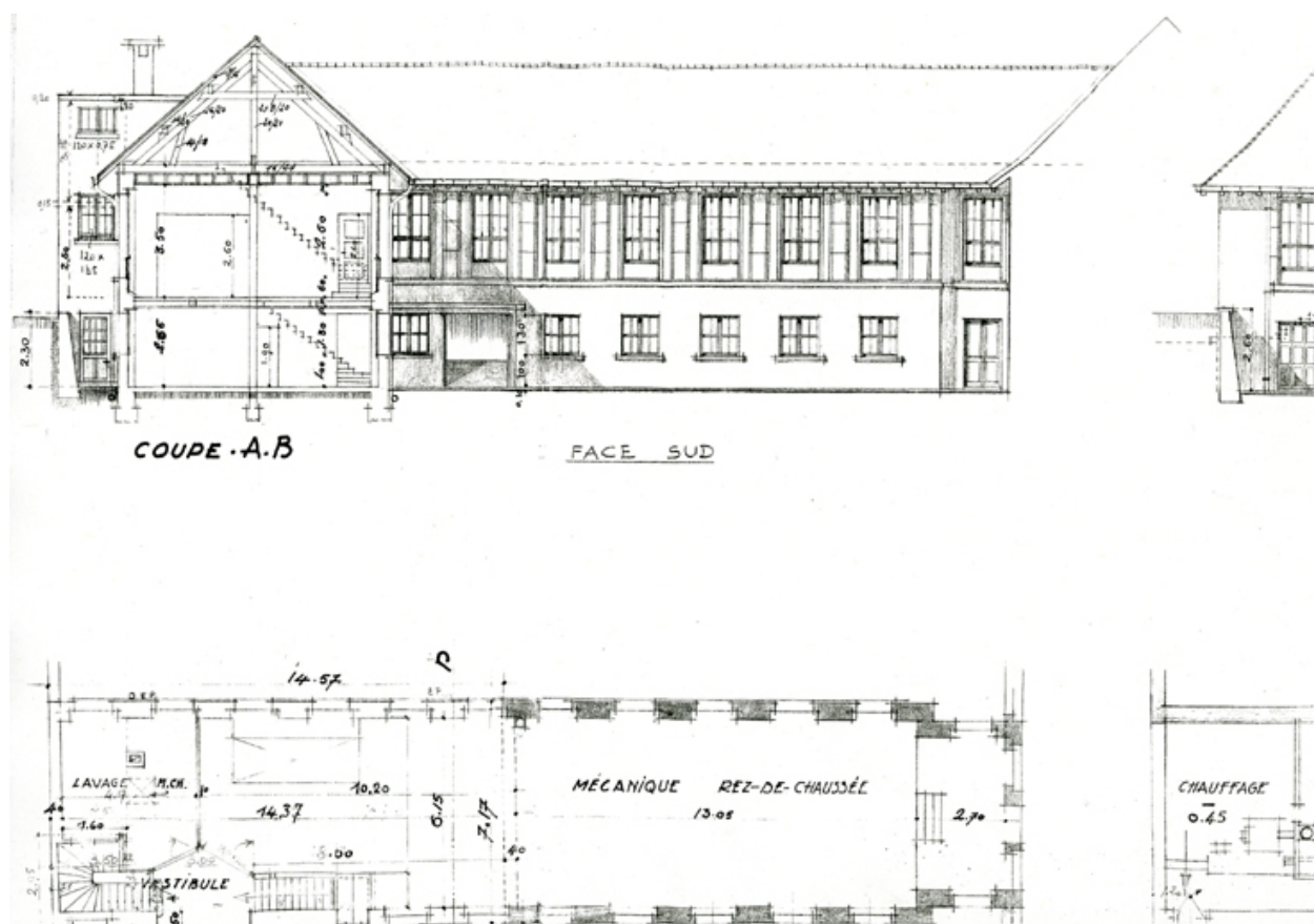
Coupe façade sud
