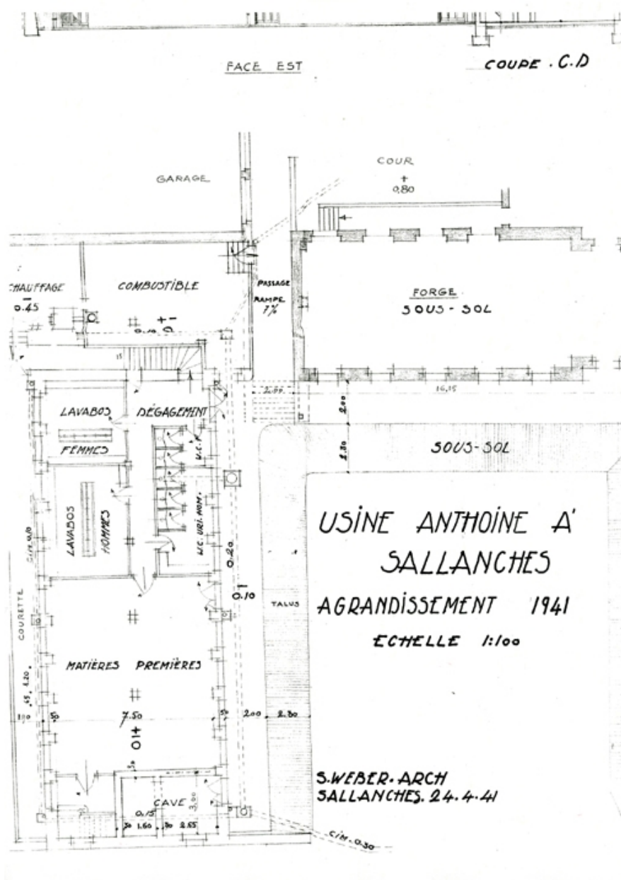
Plan masse 1941 : agrandissement de l'usine Anthoine
