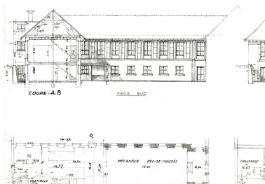
Coupe façade sud Phot. Nadine Halitim-Dubois IVR82_20057400016NUC
