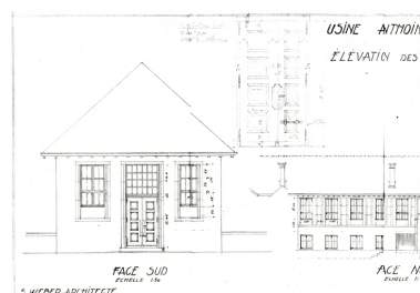
Elévation façade sud (Weber architecte) Phot. Nadine Halitim-Dubois IVR82_20057400014NUC
