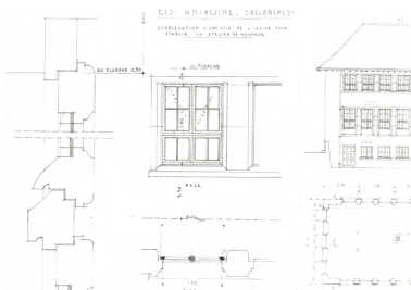
Surélévation d'une aile de l'usine pour établir un atelier de montage Phot. Nadine Halitim-Dubois IVR82_20057400019NUC
