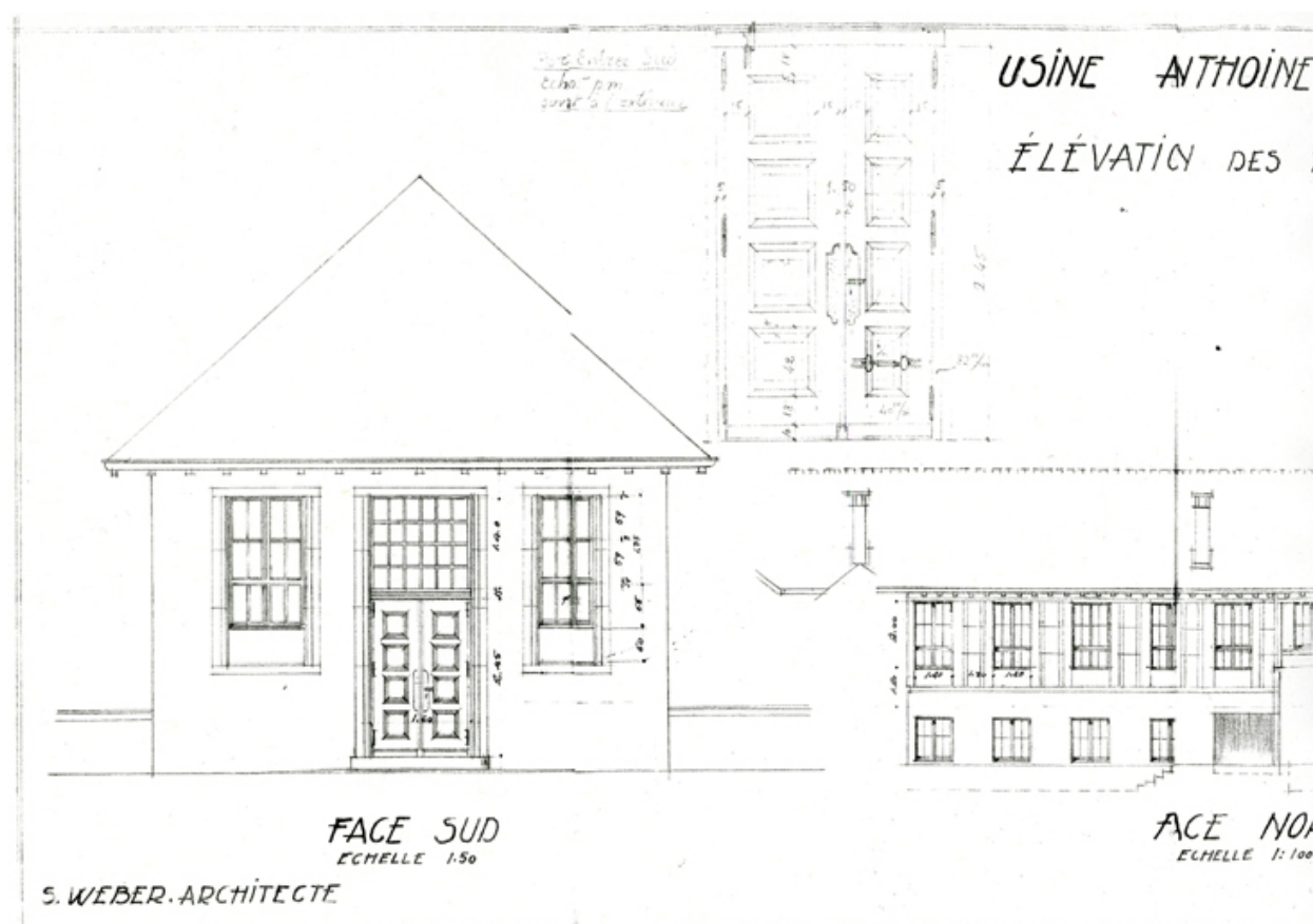
Elévation façade sud (Weber architecte)
