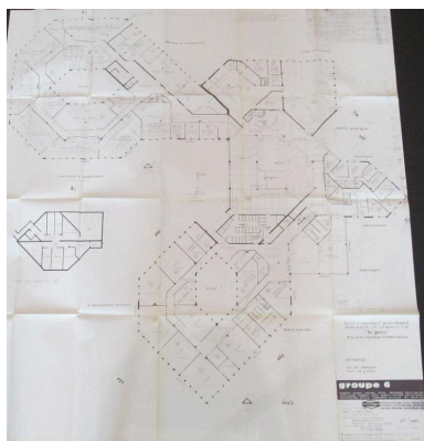
Plan de l'externat, rez-de-chaussée, Juin 1978 (AN 19910237/11). Autr. Groupe 6 (cabinet d'architecture), Repro. Valérie Pamart IVR84_20203800024NUCB
