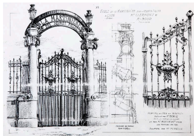
Le portail : élévation et coupes des colonnes, par F. Clermont (AC Lyon, 3 SAT 55)
