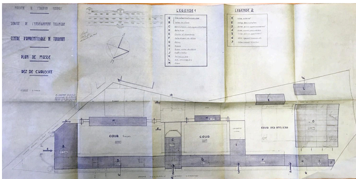
Plan de masse, rez-de-chaussée, par M. Frappa, 1950 (AD Ardèche, 2169 W 68)
