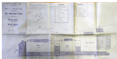
Plan de masse, rez-de-chaussée, par M. Frappa, 1950 (AD Ardèche, 2169 W 68) Autr. Maurice Frappa, Repro. Catherine Guégan IVR84_20220700171NUCA
