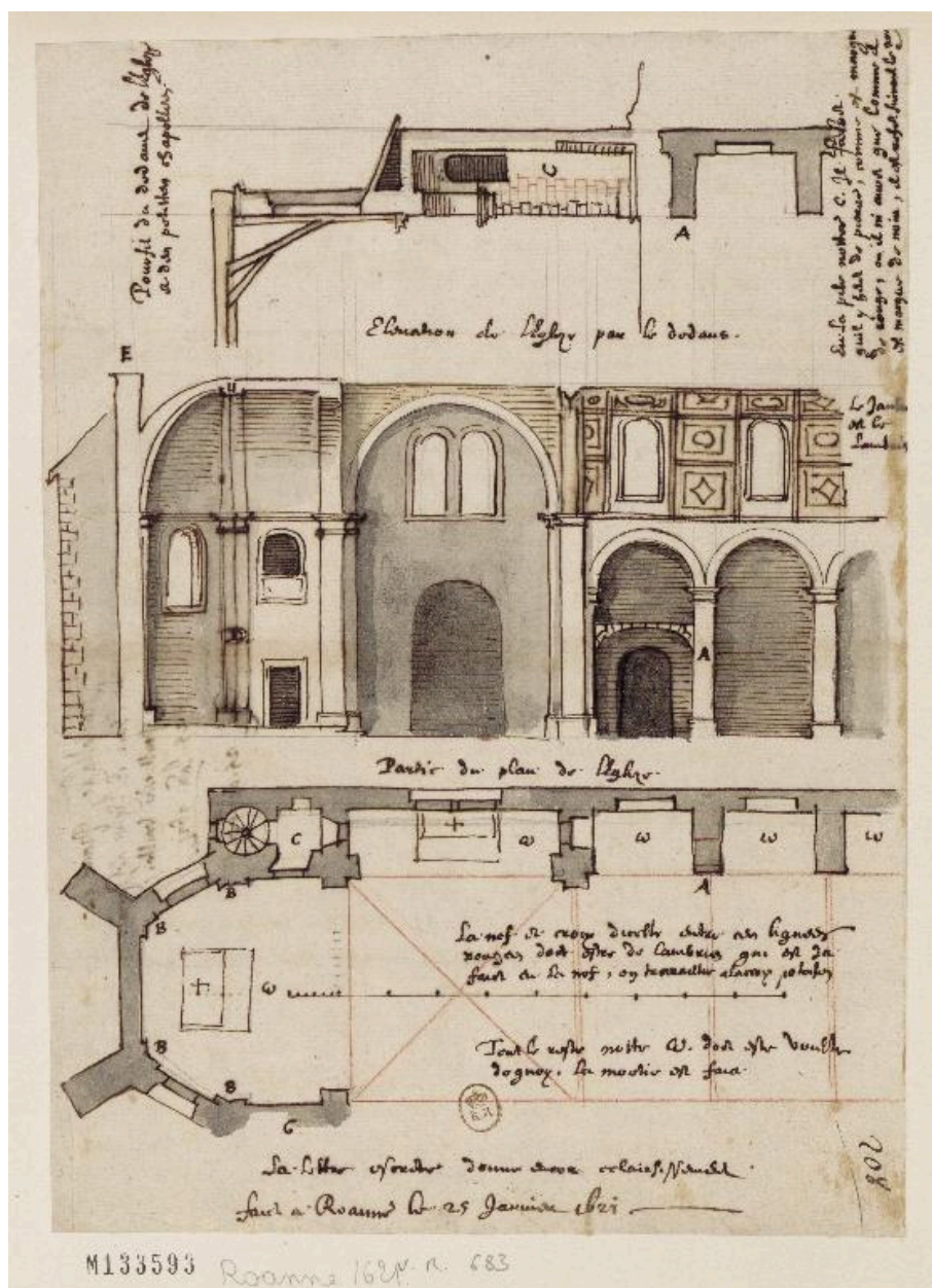
Collège de Roanne : plan partiel et coupes de l'église, le 25 Janvier 1621. B.n.F., Est. (Vallery-Radot ; 683)
