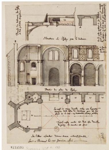
Collège de Roanne : plan partiel et coupes de l'église, le 25 Janvier 1621. B.n.F., Est. (Vallery-Radot ; 683) Autr. Etienne Martellange frère IVR82_20134201071NUCAB
