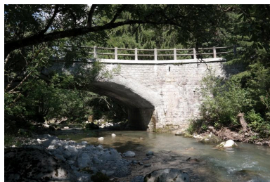
Pont de la Solitude, vue de la face amont Phot. Pascale Renard IVR84_20207401036NUCA
