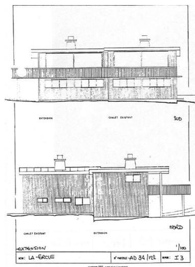
Extension. Elévations sud et nord Phot. Jean-François Lyon-Caen IVR82_20087302200NUC
