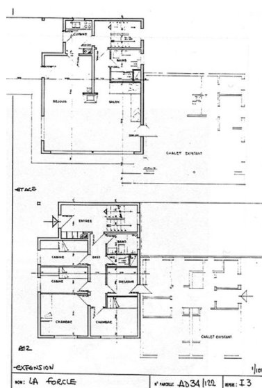
Extension. Plans du rez-de-chaussée et de l'étage Phot. Jean-François Lyon-Caen IVR82_20087302199NUC
