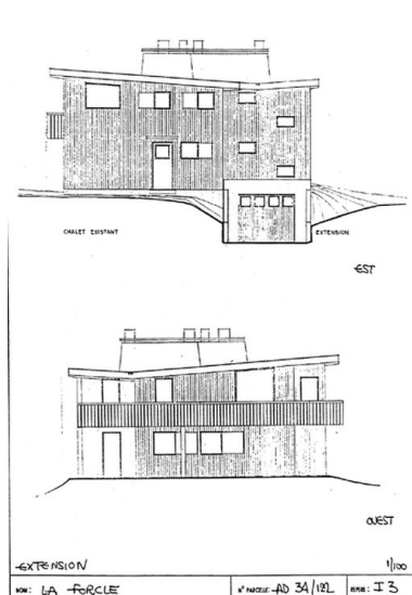
Extension. Elévations est et ouest Phot. Jean-François Lyon-Caen IVR82_20087302201NUC
