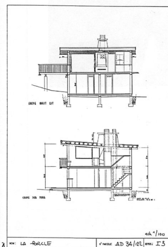
Coupes Phot. Jean-François Lyon-Caen IVR82_20087302196NUC
