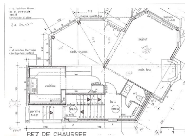
Plan du rez-de-chaussée / J.-J. Orzoni, 1982 Phot. Jean-François Lyon-Caen, Phot. C. Salomon-Pelen, Autr. Orzoni Jean-Jacques (architecte) IVR82_20087400158NUC
