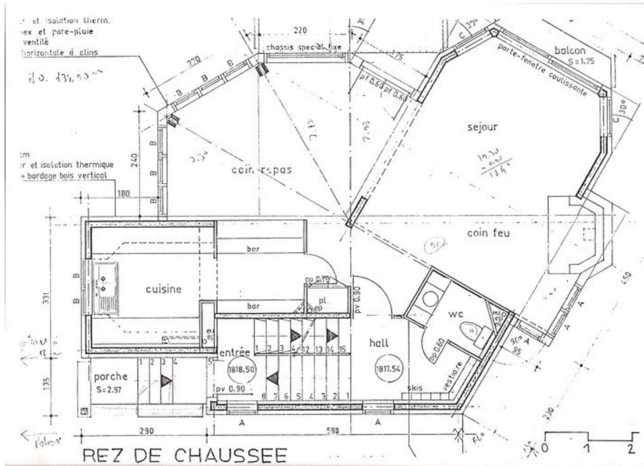
Plan du rez-de-chaussée / J.-J. Orzoni, 1982
