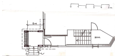
Plan de l'entrée. Projet / J.-J. Orzoni, 1991 (A. privées J. Labro) Phot. Jean-François Lyon-Caen, Phot. C. Salomon-Pelen, Autr. Orzoni Jean-Jacques (architecte)
