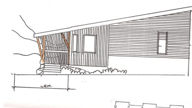
Projet de porche d'entrée. Elévation / J.-J. Orzoni, 1991 (A. privées J. Labro)
