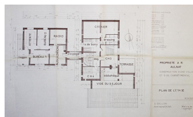
Aulnat, la maison R., plan de l'étage, Gilles Gallon architecte, décembre 1970 (archives municipales d'Aulnat). Repro. Christophe Laurent, Autr. Gilles GALLON IVR84_20246301826NUCA
