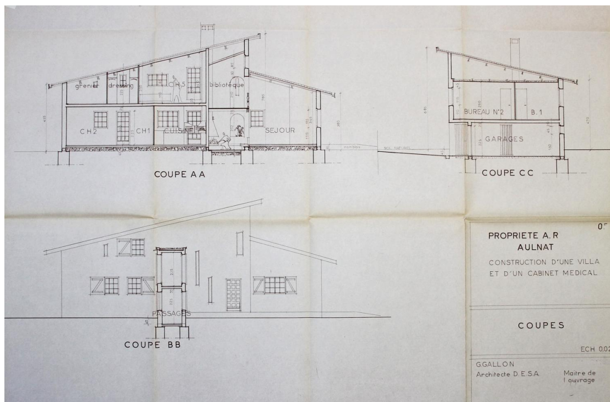
Aulnat, la maison R., coupes, Gilles Gallon architecte, décembre 1970 (archives municipales d'Aulnat).
