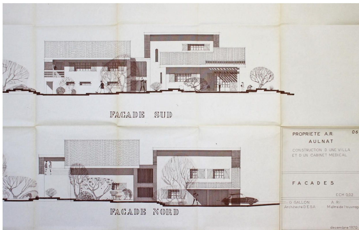
Aulnat, la maison R., façades nord et sud, Gilles Gallon architecte, décembre 1970 (archives municipales d'Aulnat).
