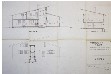
Aulnat, la maison R., coupes, Gilles Gallon architecte, décembre 1970 (archives municipales d'Aulnat). Repro. Christophe Laurent, Autr. Gilles GALLON IVR84_20246301828NUCA
