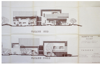
Aulnat, la maison R., façades nord et sud, Gilles Gallon architecte, décembre 1970 (archives municipales d'Aulnat). Repro. Christophe Laurent, Autr. Gilles GALLON IVR84_20246301827NUCA
