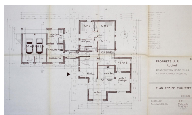
Aulnat, la maison R., plan du rez-de-chaussée, Gilles Gallon architecte, décembre 1970 (archives municipales d'Aulnat). Repro. Christophe Laurent, Autr. Gilles GALLON IVR84_20246301825NUCA
