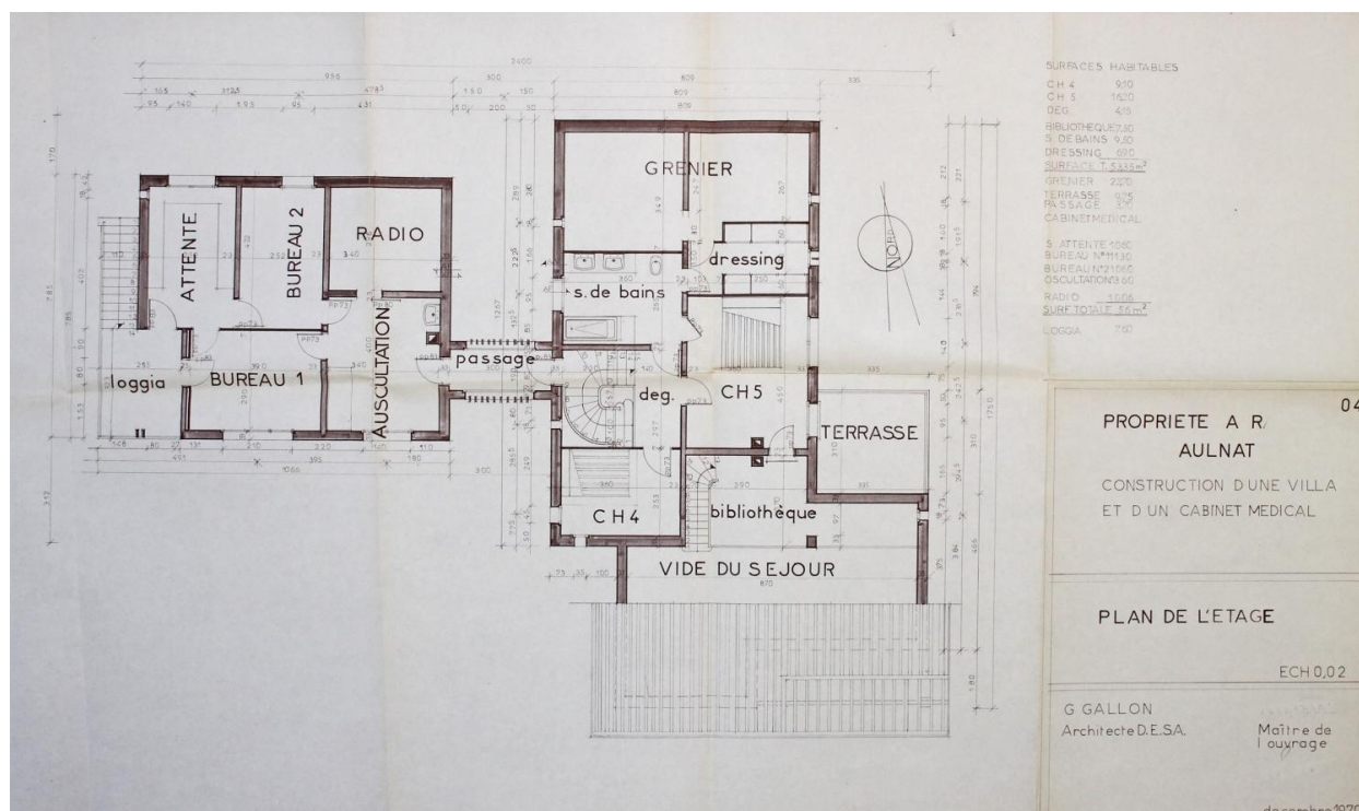
Aulnat, la maison R., plan de l'étage, Gilles Gallon architecte, décembre 1970 (archives municipales d'Aulnat).
