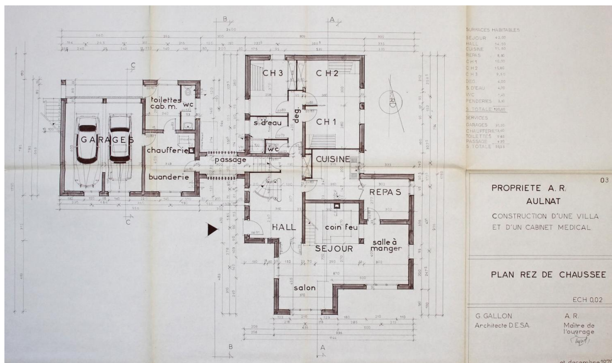
Aulnat, la maison R., plan du rez-de-chaussée, Gilles Gallon architecte, décembre 1970 (archives municipales d'Aulnat).
