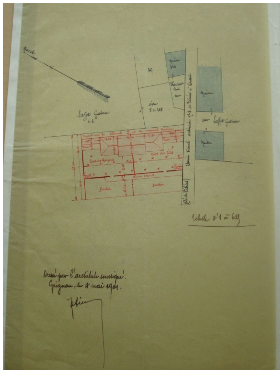
Commune de Rousset. Construction d'un groupe scolaire. Plan de l'emplacement, par Auguste Etienne, 1901.
