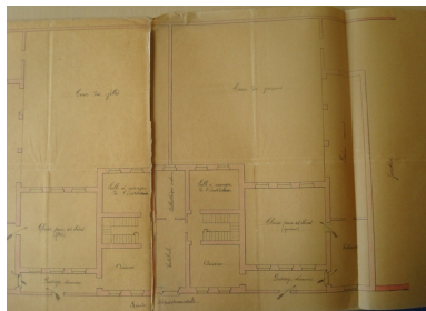
Commune de Rousset. Construction d'un groupe scolaire. Croquis sommaire, dressé le 11 novembre 1882 par (Rasclas), agent voyer d'arrondissement. Phot. Alain Franchella, Autr. agent voyer (Rasclas) IVR82_20112600100NUCA
