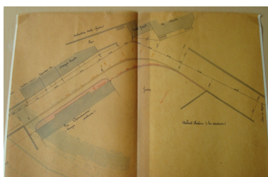
Route départementale n° 4 bis de Montélimar à Nyons. Déplacement du mur de clôture de l'école. Plan de la traverse de Rousset, dressé par l'agent voyer cantonal Reynaud, le 30 avril 1909. Détail. Phot. Alain Franchella, Autr. agent voyer cantonal Reynaud IVR82_20112600104NUCA
