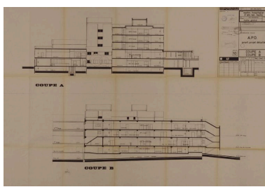
Coupe Repro. Denys Harreau IVR82_20147300764NUCB
