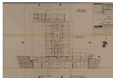
Plan du 2e étage Repro. Denys Harreau IVR82_20147300762NUCB
