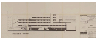
Façade nord Repro. Denys Harreau IVR82_20147300767NUCB
