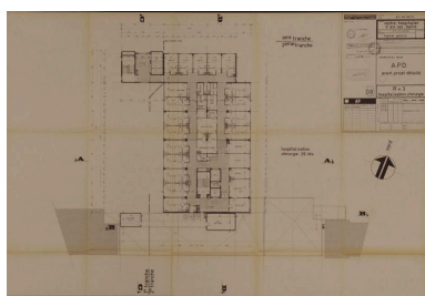
Plan du 3e étage Repro. Denys Harreau IVR82_20147300763NUCB
