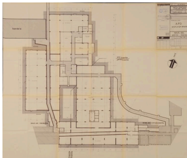
Plan des sous-sols Repro. Denys Harreau IVR82_20147300774NUCB
