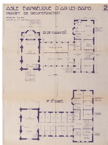
Plans du rez-de-chaussée et du 1er étage Repro. François Fouger IVR82_20067300060NUCB
