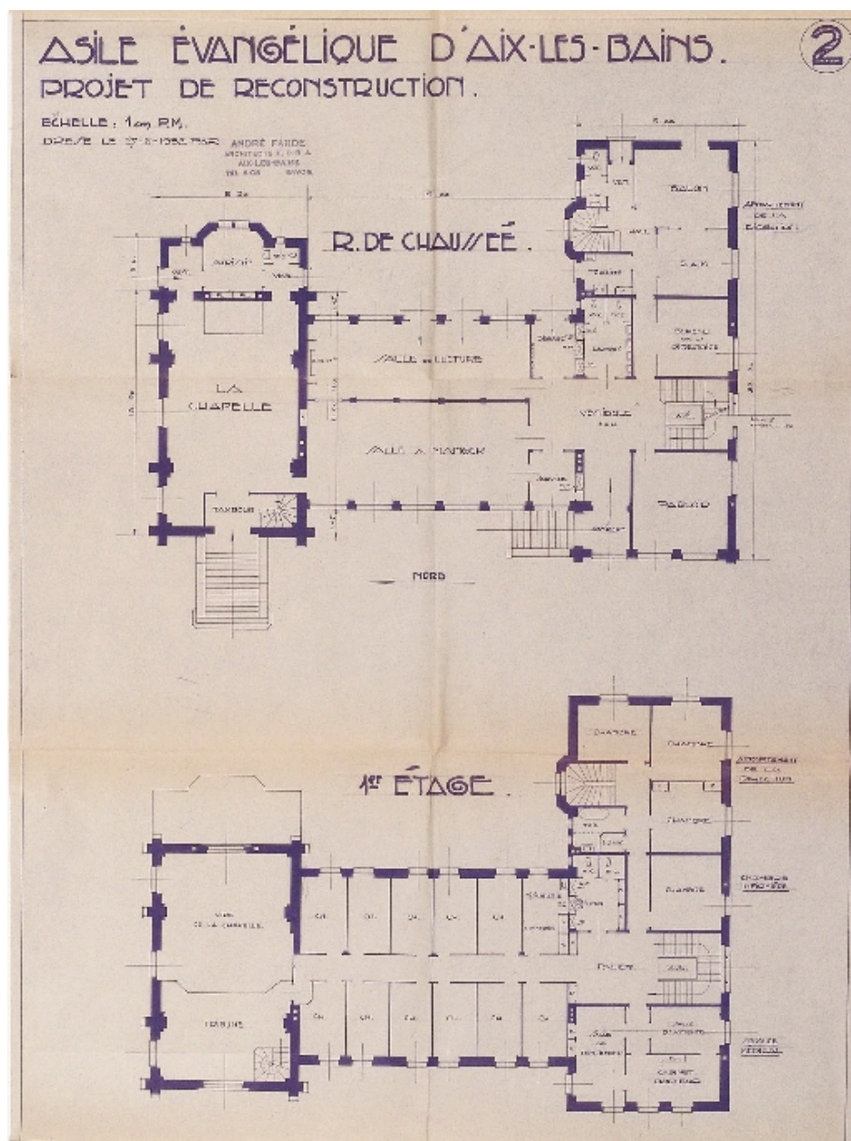
Plans du rez-de-chaussée et du 1er étage
