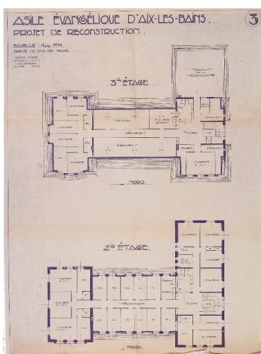
Plans des 2e et 3e étages Repro. François Fouger IVR82_20067300061NUCB
