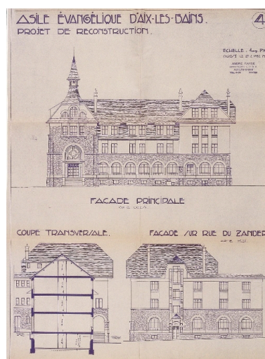
Coupe et élévation Repro. François Fouger IVR82_20067300059NUCB
