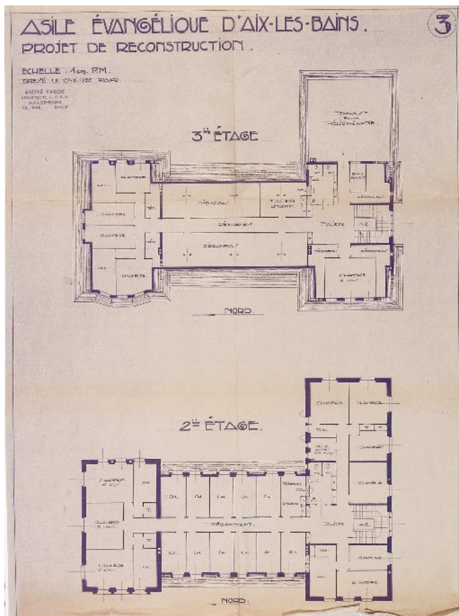
Plans des 2e et 3e étages
