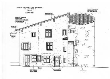
Façade est. Phot. Caroline Guibaud, Autr. Jacques Porte IVR82_20134201543NUC
