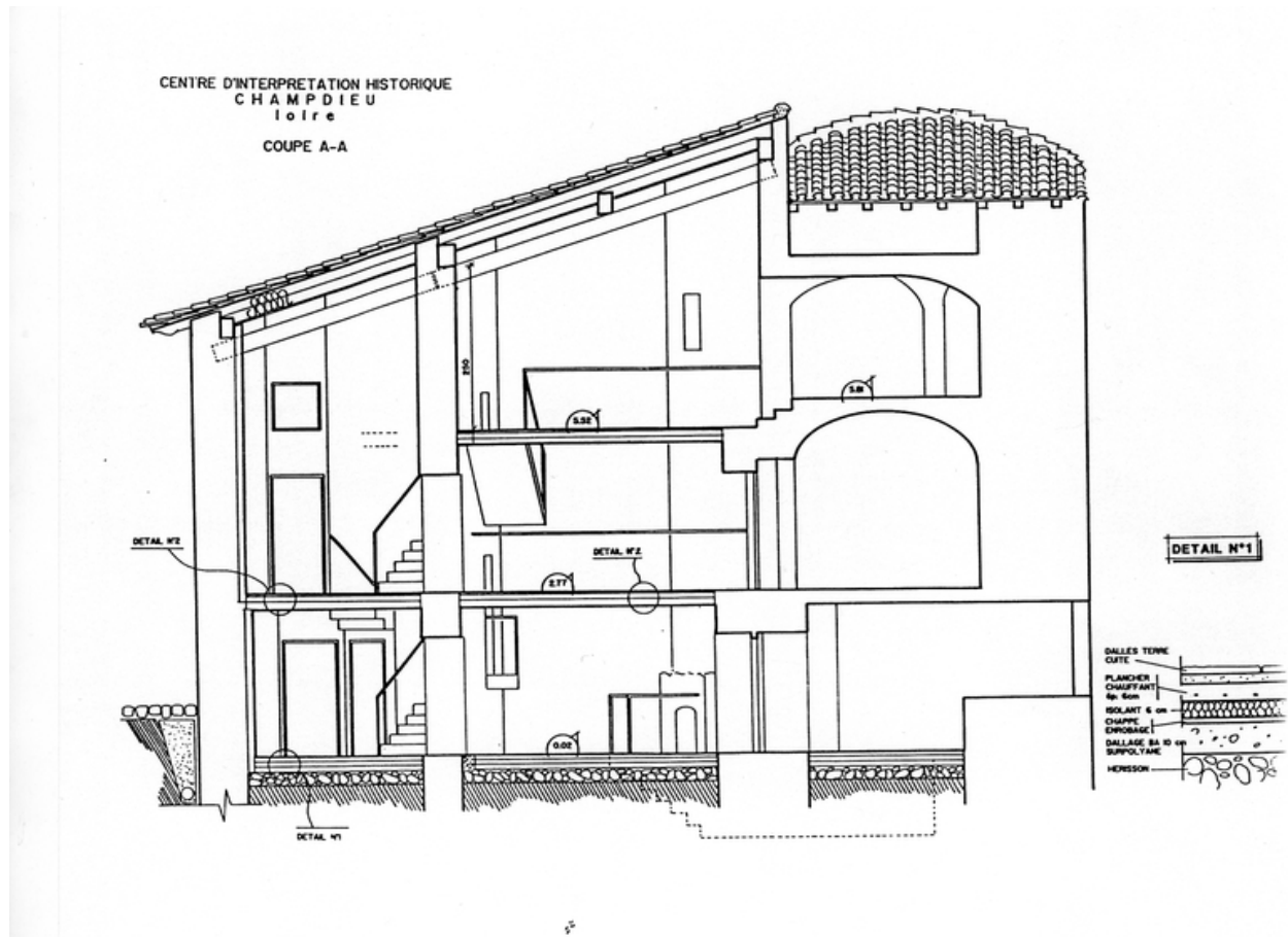
Coupe A-A.
