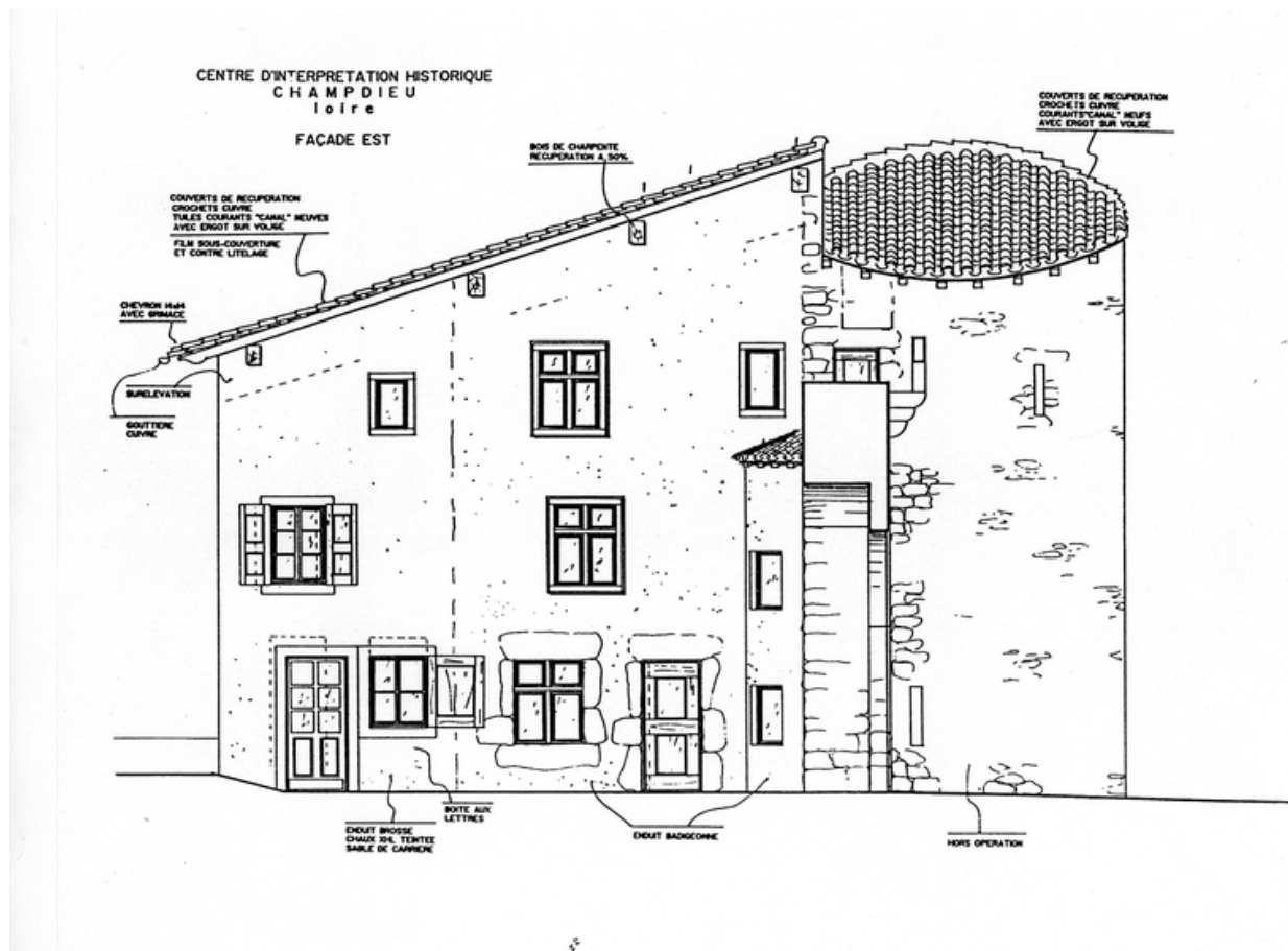
Façade est.
