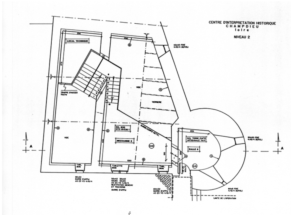
[Plan du] Niveau 2.
