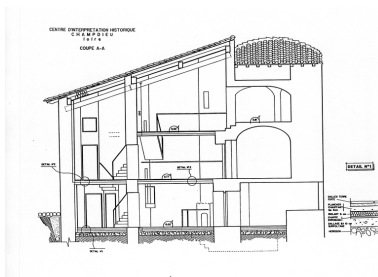
Coupe A-A. Phot. Caroline Guibaud, Autr. Jacques Porte IVR82_20134201544NUC
