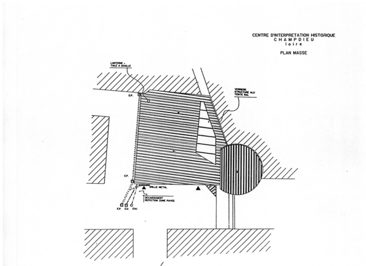
Plan masse [et de toiture].
