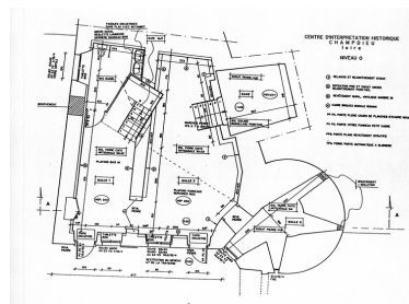
[Plan du] Niveau 0. Phot. Caroline Guibaud, Autr. Jacques Porte IVR82_20134201539NUC
