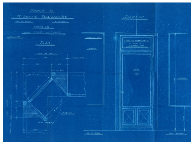
Plan et élévation de la porte d'entrée du magasin Repro. François Fouger IVR82_20057302084NUCB
