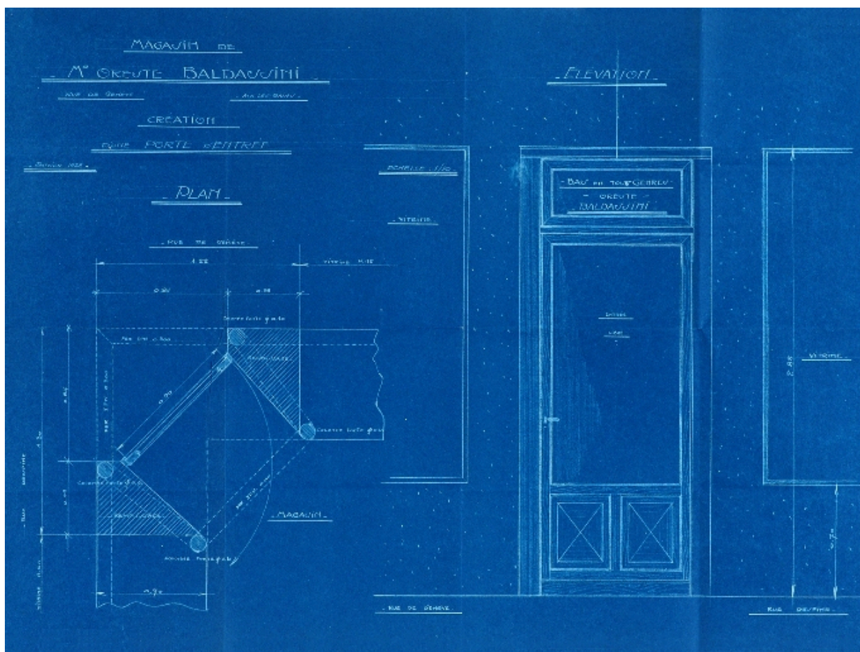
Plan et élévation de la porte d'entrée du magasin
