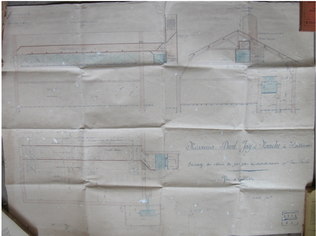
Messieurs Durel Jay et Naacke à Montbrison. Séchage à cônes de pin par aérocondenseur système Frédéric Fouché. 1908. Vue d'ensemble du document.
