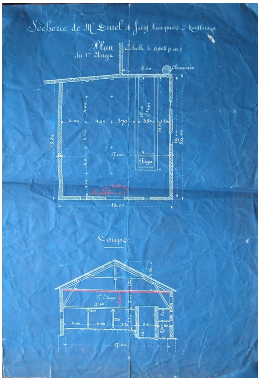
Sécherie de Mr Durel et Jay, banquiers à Montbrison. Plan du 1er étage. Coupe. 1er quart 20e siècle.
