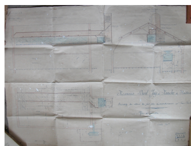
Messieurs Durel Jay et Naacke à Montbrison. Séchage à cônes de pin par aérocondenseur système Frédéric Fouché. 1908. Vue d'ensemble du document. Repro. Thierry Monnet, Autr. Frédéric (constructeur) Fouché IVR82_20134204373NUCA
