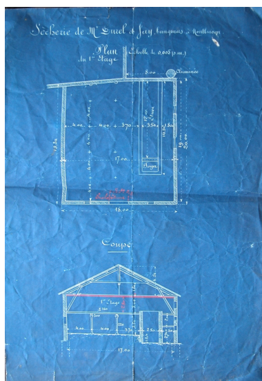
Sècherie de Mr Durel et Jay, banquiers à Montbrison. Plan du 1er étage. Coupe. 1er quart 20e siècle. Repro. Thierry Monnet IVR82_20134204372NUCA
