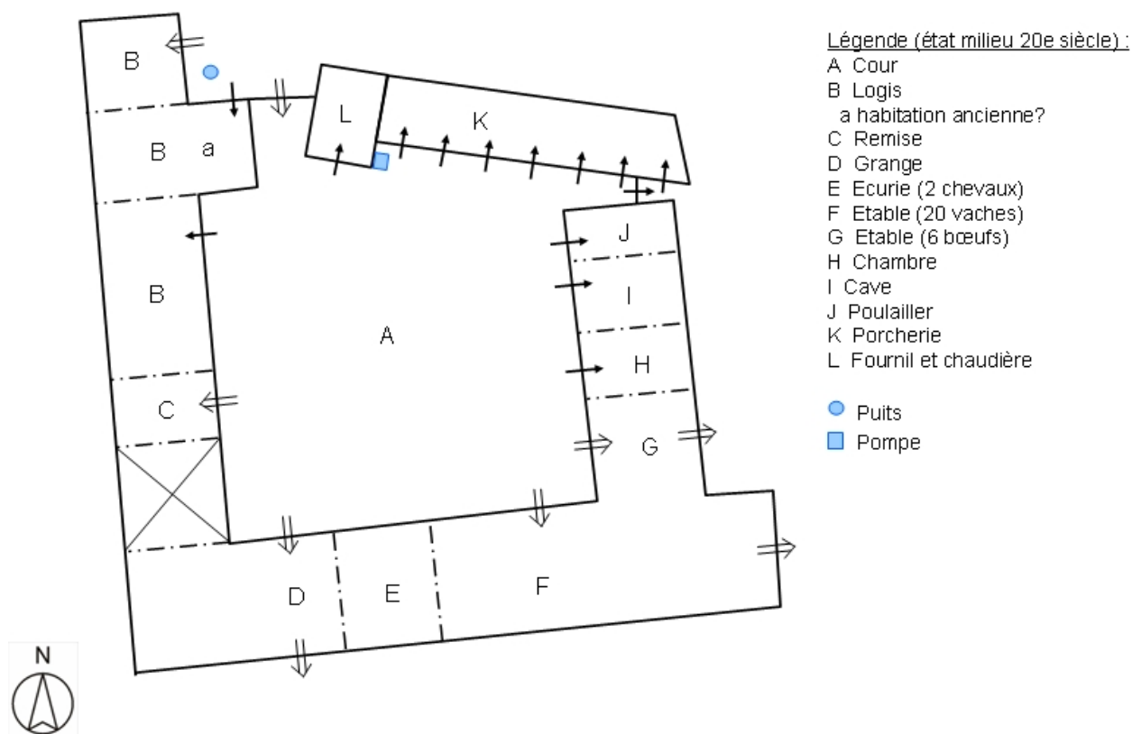
Plan-masse.
