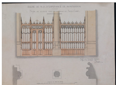
Eglise de N. D. D'Espérance de Montbrison. Projet de clôture pour la chapelle du Sacré-Coeur Phot. Eric Dessert, Autr. Claudius Jamot IVR82_20104200449NUCA
