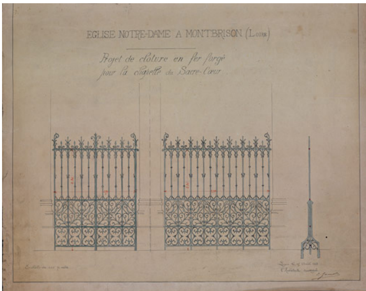
Eglise Notre-Dame à Montbrison (Loire). Projet de clôture en fer forgé pour la chapelle du Sacré-Coeur.
