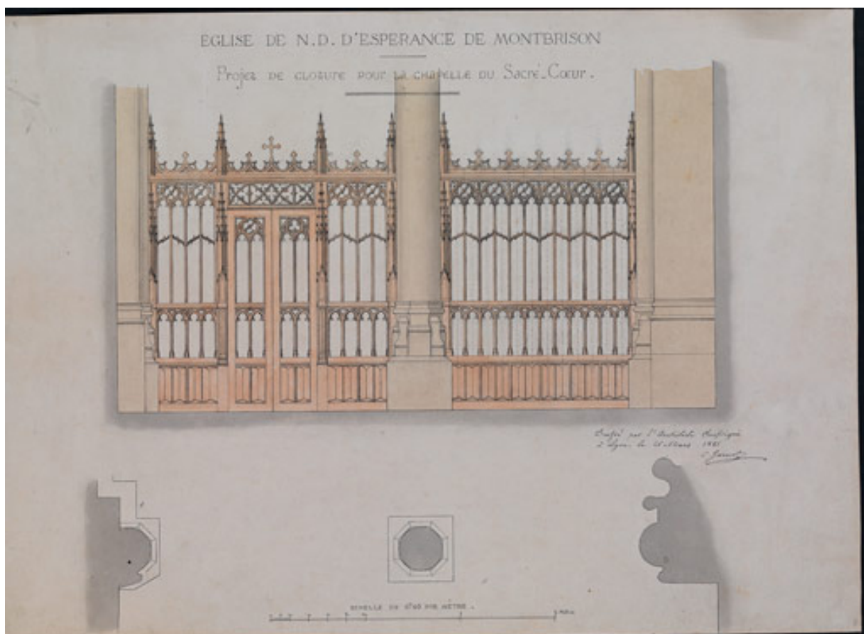
Eglise de N. D. D'Espérance de Montbrison. Projet de clôture pour la chapelle du Sacré-Coeur
