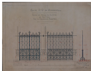
Eglise N-D de Montbrison (Loire). Projet de grille de clôture en fer forgé pour la chapelle du Sacré-Coeur. Phot. Eric Dessert, Autr. Claudius Jamot IVR82_20104200451NUCA
