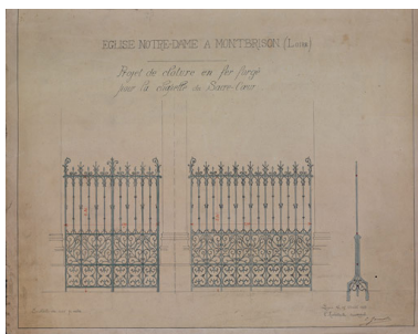
Eglise Notre-Dame à Montbrison (Loire). Projet de clôture en fer forgé pour la chapelle du Sacré-Coeur. Phot. Eric Dessert, Autr. Claudius Jamot IVR82_20104200448NUCA
