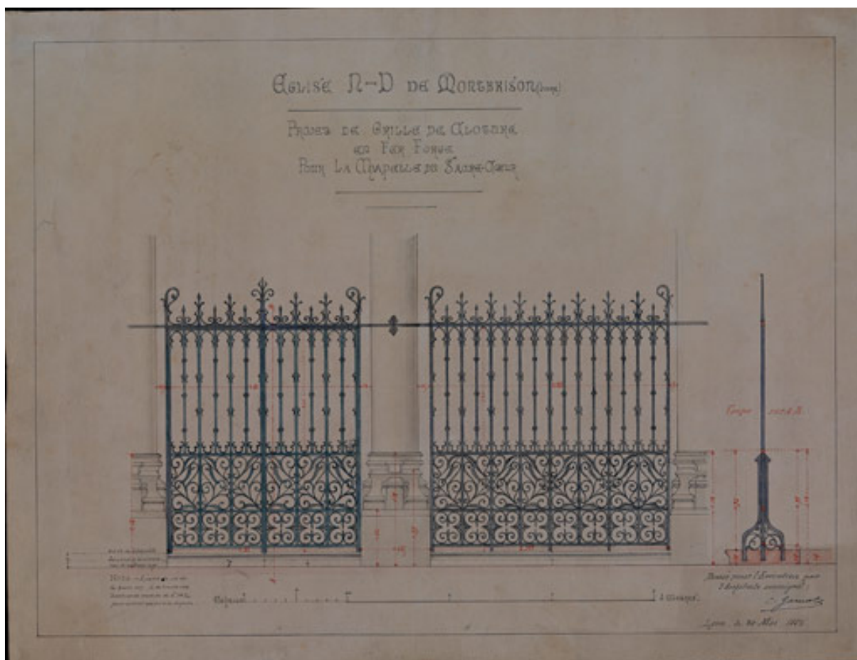
Eglise N-D de Montbrison (Loire). Projet de grille de clôture en fer forgé pour la chapelle du Sacré-Coeur.
