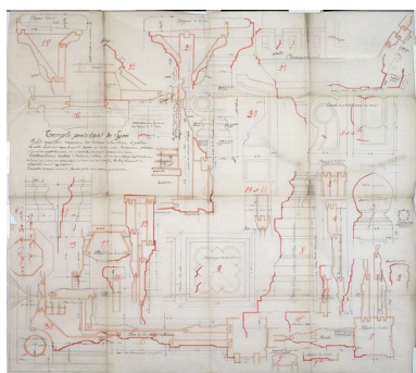
Profil grandeur d'exécution des boiseries de la chaire à prêcher. Repro. Didier Gourbin, Autr. Gaspard André IVR82_20106906103NUCA
