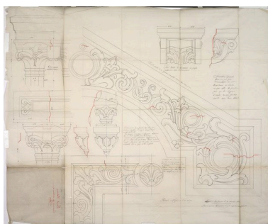
Dessin d'exécution pour les boiseries de la chaire. Repro. Didier Gourbin, Autr. Gaspard André IVR82_20106906114NUCA
