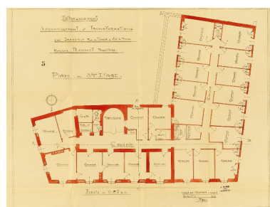
Plan du 3e étage Repro. François Fouger IVR82_20087300149NUCB
