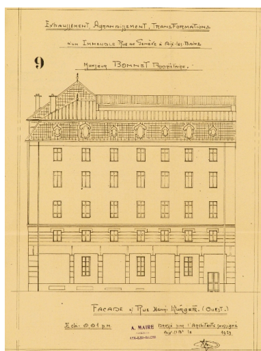
Elévation ouest Repro. François Fouger IVR82_20087300153NUCB
