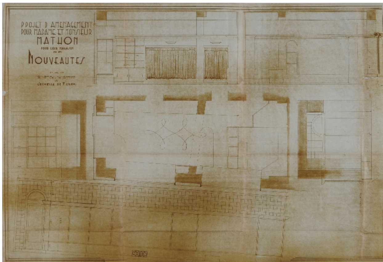
Plan perspectif du magasin
