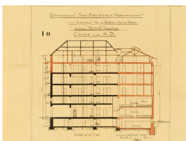
Coupe est-ouest Repro. François Fouger IVR82_20087300154NUCB
