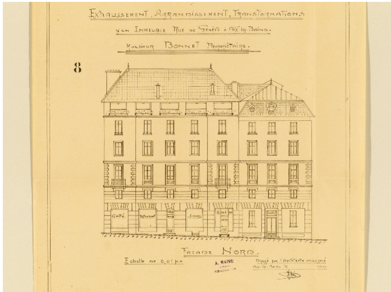
Elévation nord
