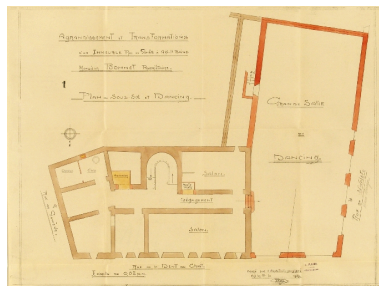
Plan du sous-sol Repro. François Fouger IVR82_20087300145NUCB
