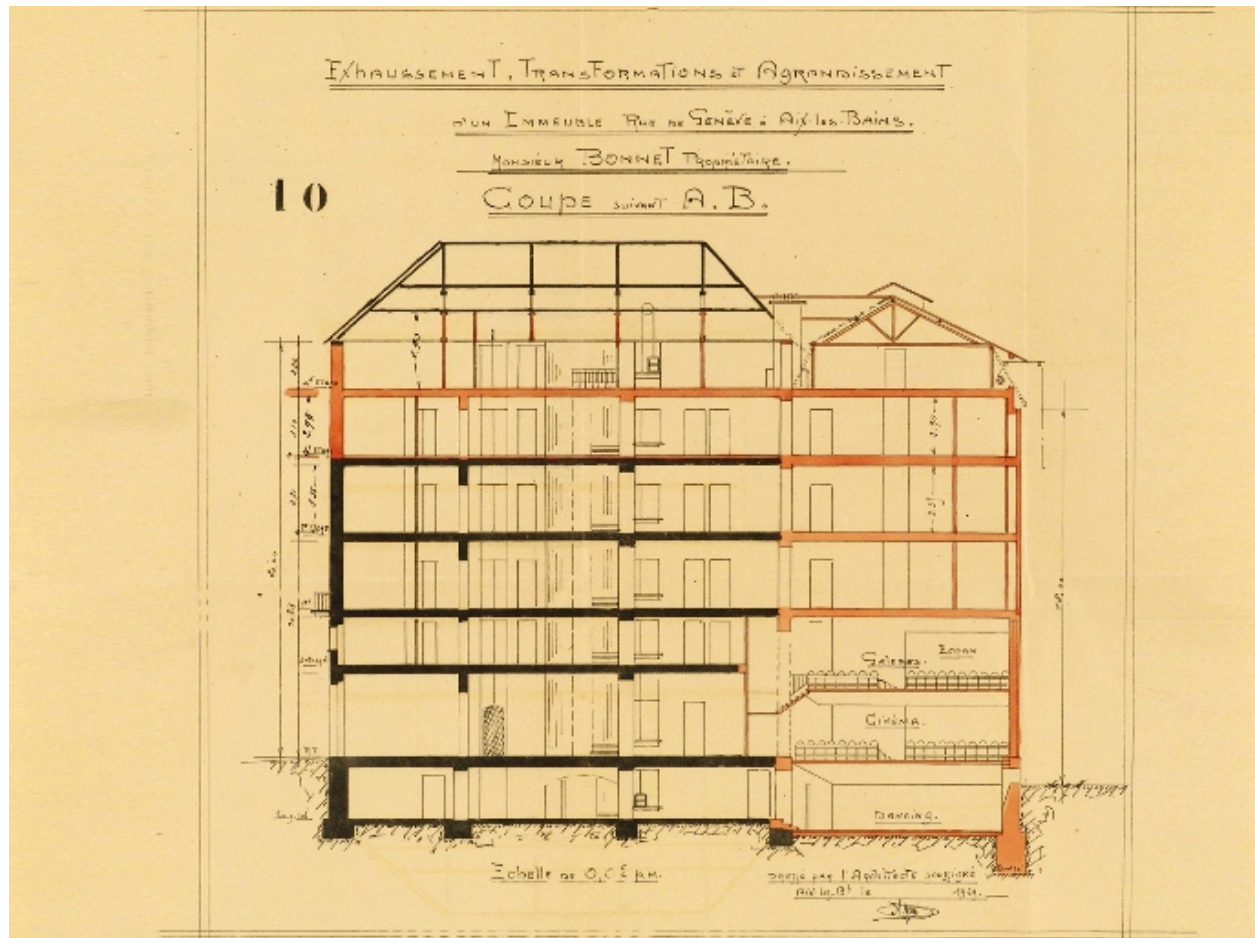
Coupe est-ouest
