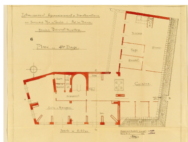
Plan du 4e étage Repro. François Fouger IVR82_20087300150NUCB
