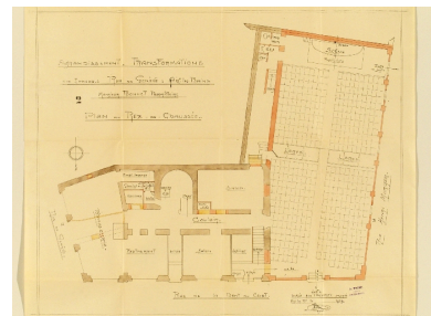
Plan du rez-de-chaussée Repro. François Fouger IVR82_20087300146NUCB
