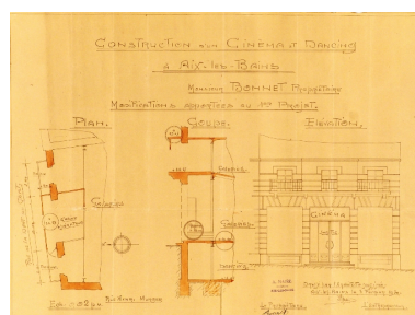
Modifications : plan, coupe et élévation Repro. François Fouger IVR82_20087300155NUCB
