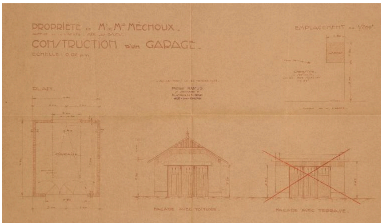
Plan et élévations du garage, 1933
