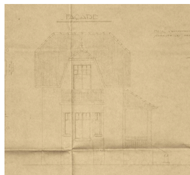
Façade sur rue, 1932 Repro. Denys Harreau IVR82_20137301120NUCB
