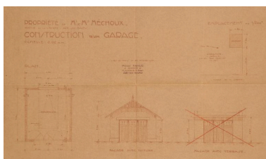
Plan et élévations du garage, 1933 Repro. Denys Harreau IVR82_20137301121NUCB
