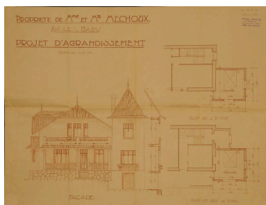
Projet d'agrandissement, plans et élévation, 1934 Repro. Denys Harreau IVR82_20137301117NUCB
