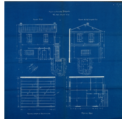
AC Lyon : 344 WP 191 PCA 300, plan, coupe, élévation de la maison de monsieur Durand par monsieur Delalande. 1925 Repro. Gilles Bernasconi IVR82_20096901839NUCA
