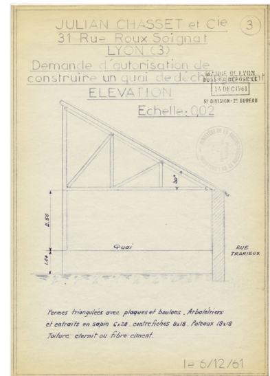
AC Lyon : 364 WP 066 PCA n° 673, élévation du quai de déchargement, Julian Chasset et Cie, 1961. Repro. Gilles Bernasconi IVR82_20096901870NUCA
