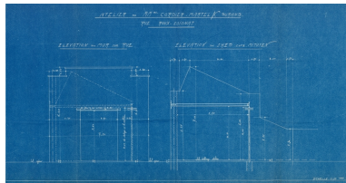
AC Lyon : 344 WP 083 PCA 0248, coupe du hangar à construire pour M.M. Cordier, Durand et Martel par M. Pinet architecte, 1920. Repro. Gilles Bernasconi IVR82_20096901828NUCA
