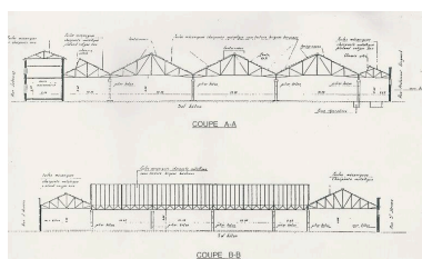
Coupes des façades du dépôt Parmentier (sources DAU Ville de Lyon) Phot. Nadine Halitim-Dubois IVR82_20116900457NUC
