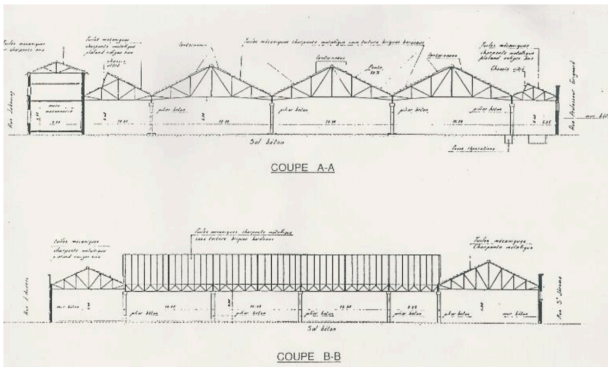
Coupes des façades du dépôt Parmentier (sources DAV Ville de Lyon)
