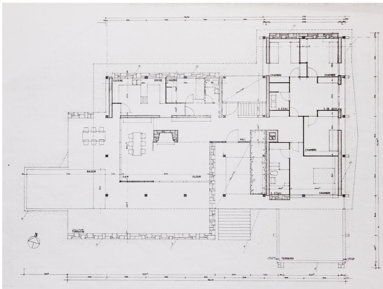
Chamalières, la Maison B., plan du rez-de-chaussée (non définitif), vers 1964, Fernand CARPENTIER architecte (archives famille Carpentier).
