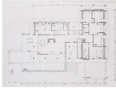
Chamalières, la Maison B., plan du rez-de-chaussée (non définitif), vers 1964, Fernand CARPENTIER architecte (archives famille Carpentier). Repro. Christophe Laurent, Autr. Fernand Carpentier IVR84_20216302422NUCA
