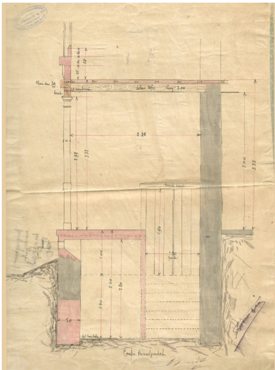
Coupe transversale sur l'extension
