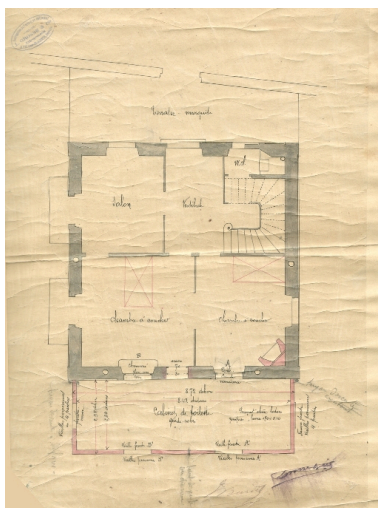
Plan du rez-de-chaussée surélevé Repro. François Fouger IVR82_20087300385NUCB
