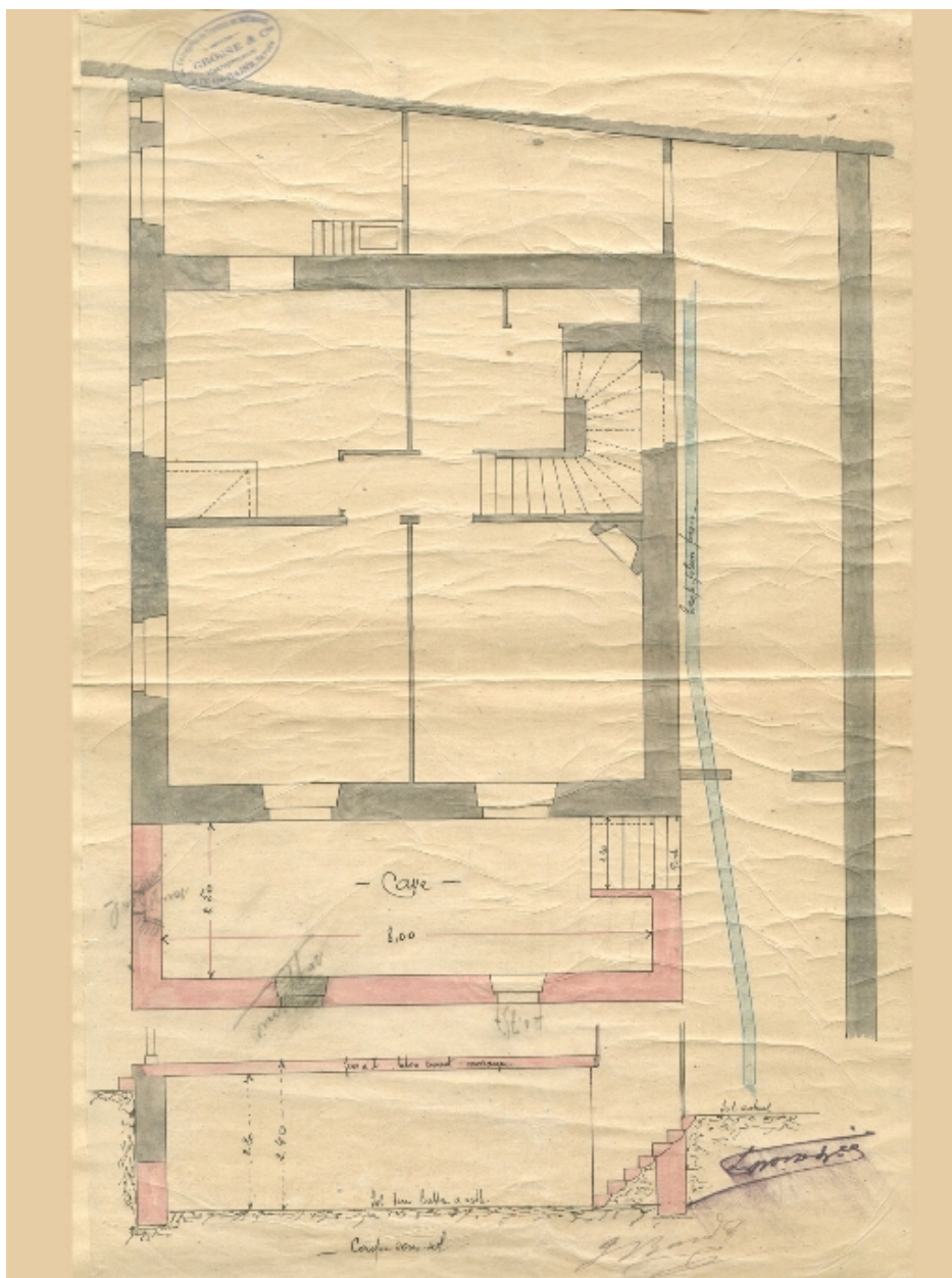
Plan et coupe du sous-sol
