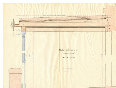
Coupe sur la véranda Repro. François Fouger IVR82_20087300389NUCB
