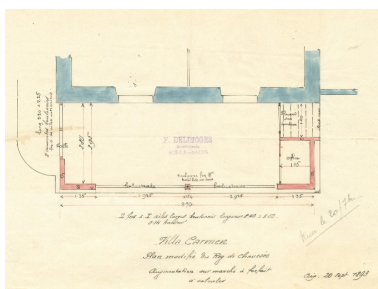
Plan de la véranda Repro. François Fouger IVR82_20087300388NUCB
