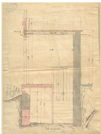
Coupe transversale sur l'extension Repro. François Fouger IVR82_20087300386NUCB
