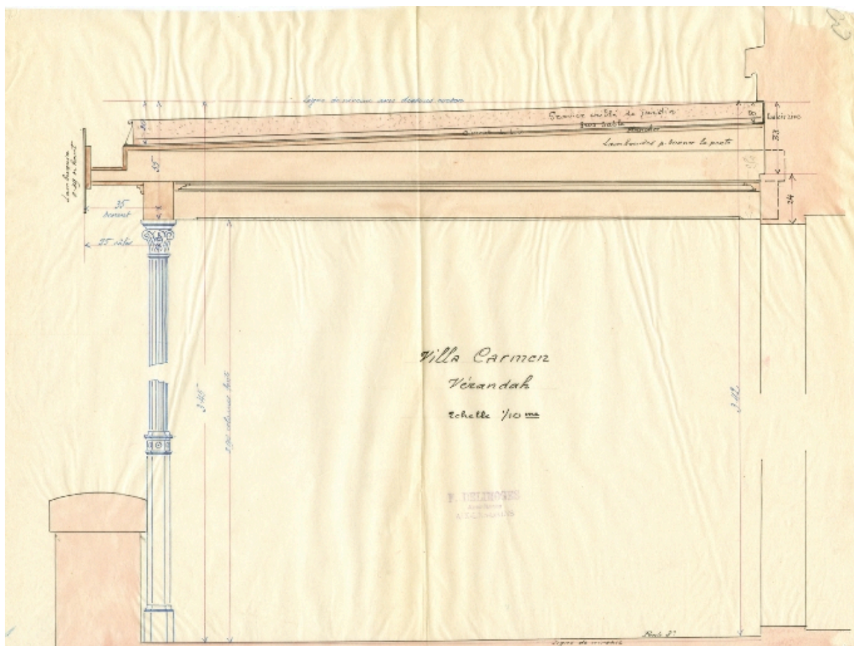
Coupe sur la véranda
