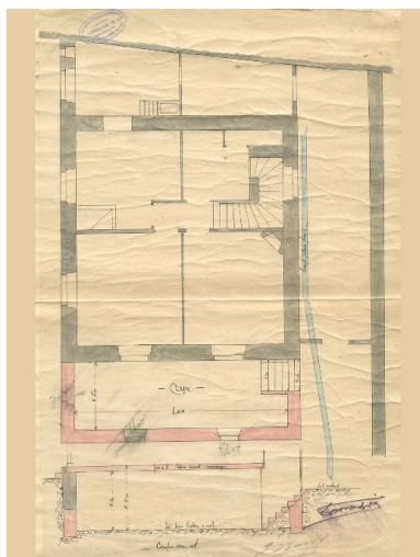
Plan et coupe du sous-sol Repro. François Fouger IVR82_20087300387NUCB
