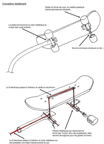
Schéma de conception. Autr. Julien Amouroux IVR84_20202600016NUCAB
