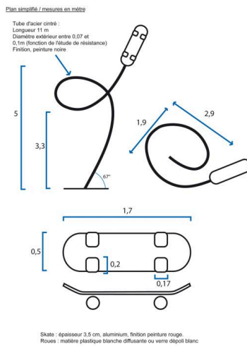
Plan simplifié, mesures en mètres. Autr. Julien Amouroux IVR84_20202600017NUCAB
