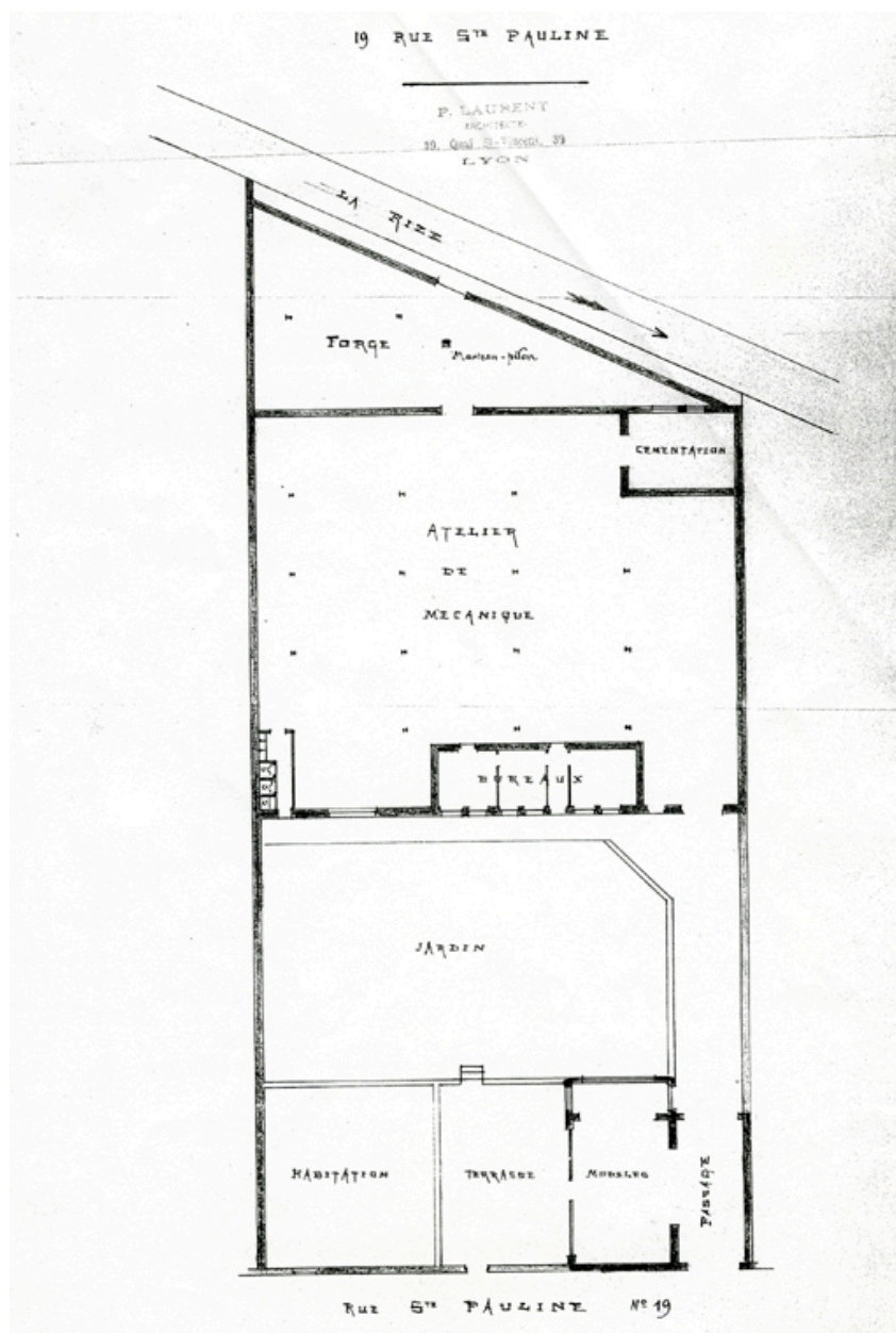
Plan des ateliers Pionchon (AD Rhône). plan des ateliers Pionchon, P. Laurent (architecte) AD Rhône. série 5M, classé 190, 1916
