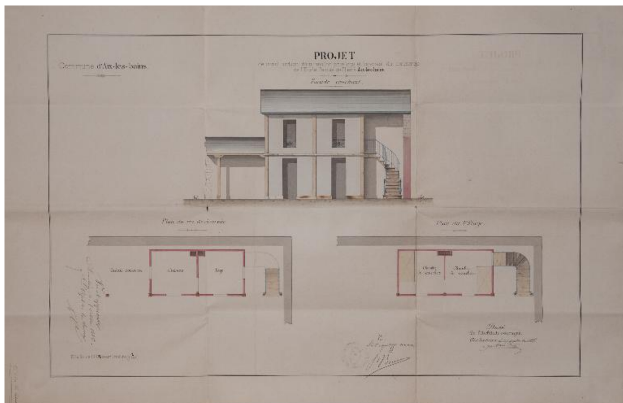
Loge de concierge, 1885 : plans et élévation
