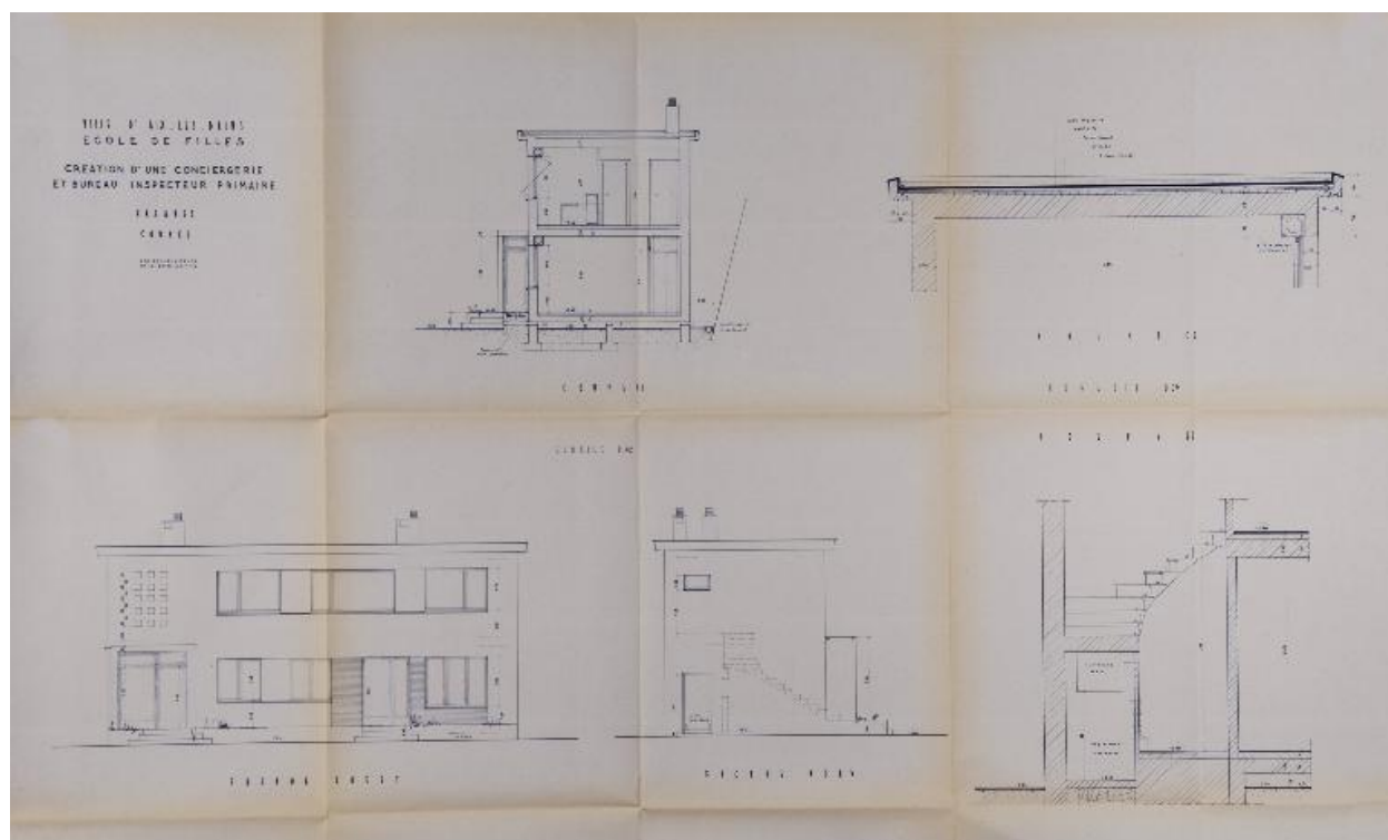
Conciergerie, 1962 : coupes et façades
