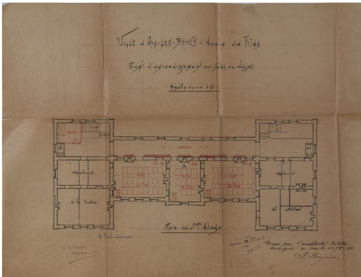
Plan du 2e étage, 1902
