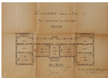
Plan du rez-de-chaussée, 1902 Repro. Denys Harreau IVR82_20157300478NUCB
