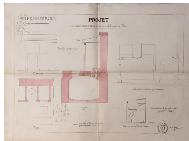
Détails, 1882 Repro. Denys Harreau IVR82_20157300483NUCB
