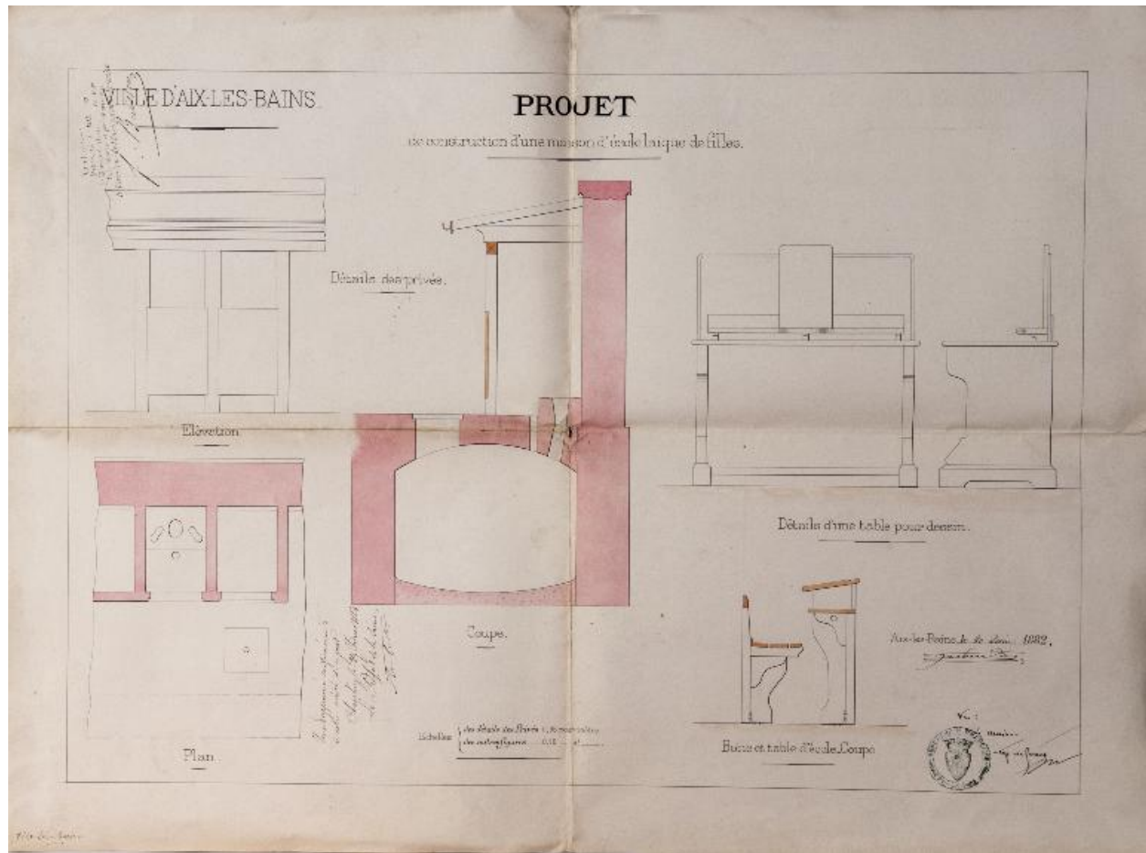
Détails d'une table à dessin et sanitaires, 1882
