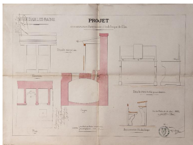
Détails d'une table à dessin et sanitaires, 1882 Repro. Denys Harreau IVR82_20157300483NUCB
