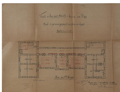
Plan du 2e étage, 1902
