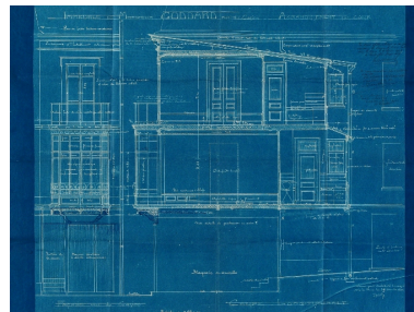
Coupe longitudinale et façade rue du Casino Repro. François Fouger IVR82_20057300227NUCB
