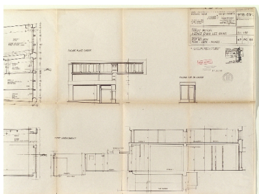
Coupes Repro. François Fouger IVR82_20057300233NUCB
