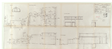
Plans et coupes Repro. François Fouger IVR82_20057300232NUCB
