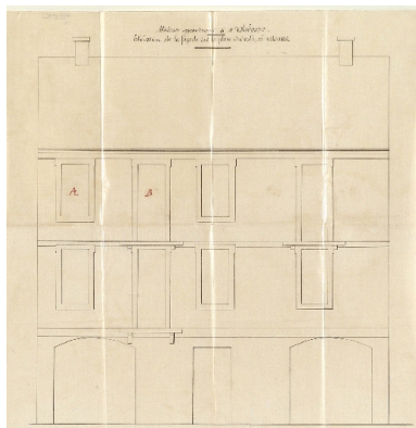
Elévation de la façade sur la place Repro. François Fouger IVR82_20057300223NUCB
