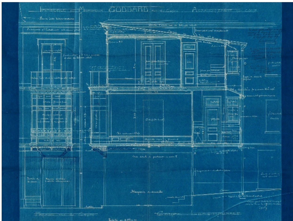
Coupe longitudinale et façade rue du Casino
