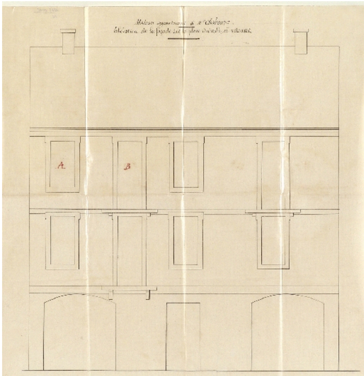
Elévation de la façade sur la place
