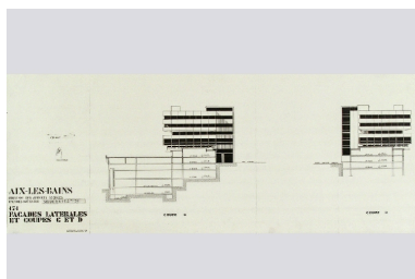
Elévations latérales Repro. François Fouger IVR82_20067300185NUCB
