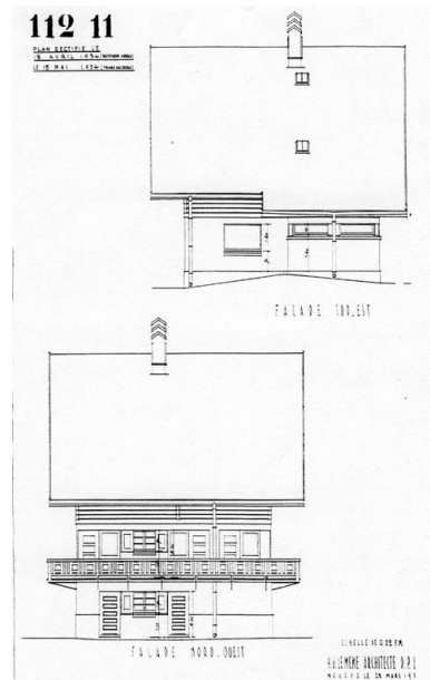
Façade sud-est et nord-ouest. N° 112-11 / Henry Jacques Le Même, 22 mars 1934, rectifié les 18 avril et 15 mai 1934 (Dossier agence n° 112) Phot. F. Véry, Autr. Le Même Henry Jacques (architecte) IVR82_20127402014NUC
