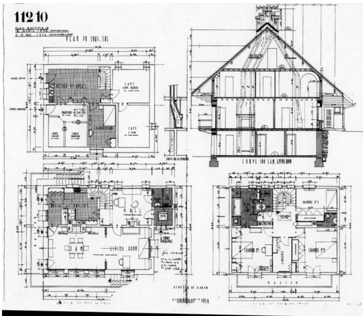
Plan du sous-sol. Plan du rez-de-chaussée. Plan du premier étage. Coupe sur S.A.M. living-room. N° 112-10 / Henry Jacques Le Même, plan rectificatif, 18 avril et 15 mai 1934 (Dossier agence n° 112)
