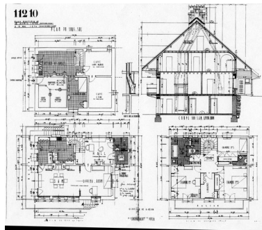
Plan du sous-sol. Plan du rez-de-chaussée. Plan du premier étage. Coupe sur S.A.M. living-room. N° 112-10 / Henry Jacques Le Même, plan rectificatif, 18 avril et 15 mai 1934 (Dossier agence n° 112) Phot. F. Véry, Autr. Le Même Henry Jacques (architecte) IVR82_20127402013NUC
