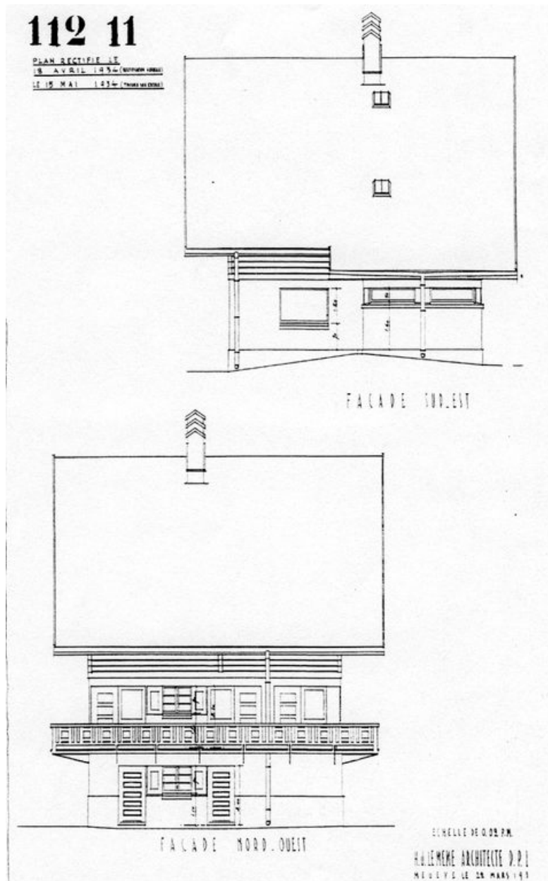
Façade sud-est et nord-ouest. N° 112-11 / Henry Jacques Le Même, 22 mars 1934, rectifié les 18 avril et 15 mai 1934 (Dossier agence n° 112)
