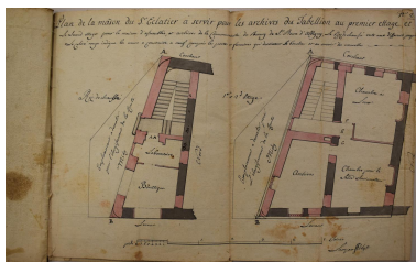
Plan de la maison du sieur Pierre Eclatier. Plan de la maison du sieur Eclatier à servir pour les archives du tabellion au premier étage... Louis Lampo (architecte). 2e feuillet : projet (AD Savoie. 138 E dépôt 30). Phot. Caroline Guibaud, Autr. Louis Lampo IVR84_20257300627NUCA
