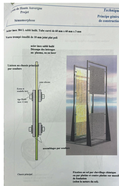
Principe général de construction (A Région Auvergne-Rhône-Alpes, 2113 WR 12) Repro. Catherine Guégan, Autr. Michel Stefanini IVR84_20241500065NUCA
