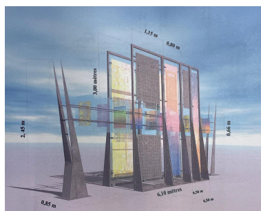
Cotation des installations (A Région Auvergne-Rhône-Alpes, 2113 WR 12) Repro. Catherine Guégan, Autr. Michel Stefanini IVR84_20241500064NUCA
