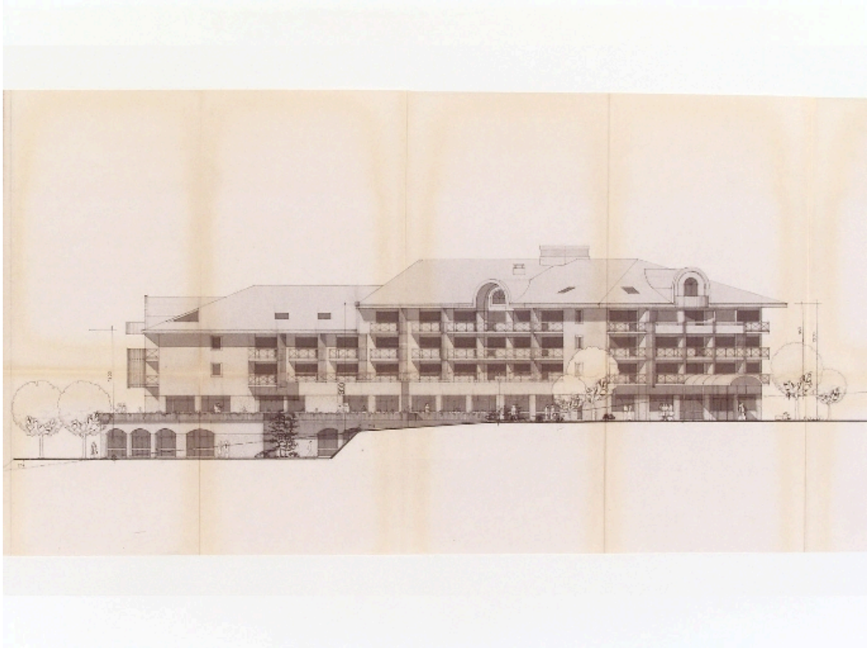
Elévation sud
