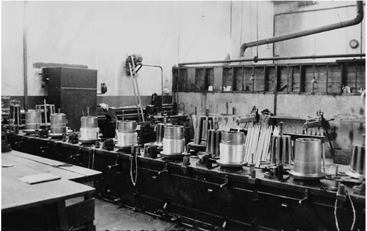
Batons de cuivre après tréfilage, dans l'atelier tréfilerie aujourd'hui désaffecté
