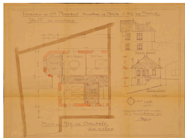
Plan du Rez-de-chaussée. Façade ouest. Façade sud Repro. Denys Harreau IVR82_20137300635NUCB
