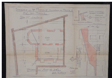
Plan sous-sol. Position de l'immeuble. Profil du terrain et fondations Repro. Denys Harreau IVR82_20137300634NUCB
