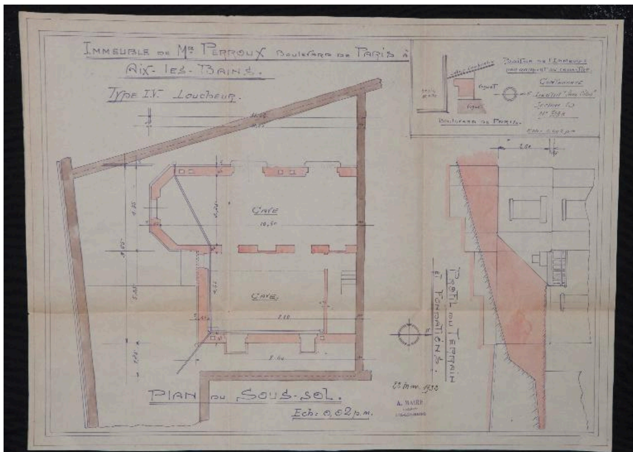
Plan sous-sol. Position de l'immeuble. Profil du terrain et fondations
