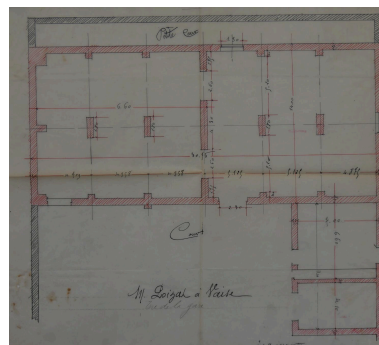
Plan usine Poizat 1894 (ACL : 314W93 - 217) Phot. Nadine Halitim-Dubois IVR84_20246900391NUCA
