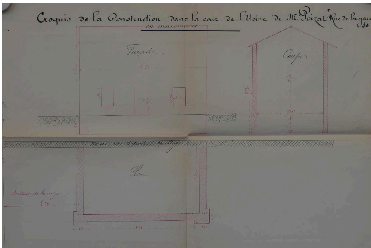
Plan usine Poizat 1890 (ACL : 314W56 - 199)
