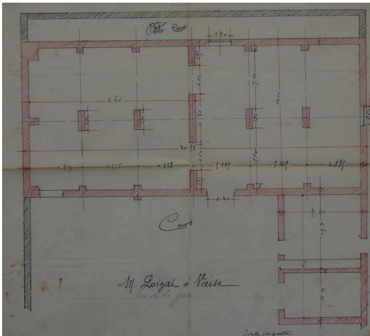
Plan usine Poizat 1894 (ACL : 314W93 - 217)
