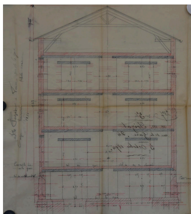
Plan usine Poizat 1894, coupe (ACL : 314W93 - 217) Phot. Nadine Halitim-Dubois IVR84_20246900392NUCA
