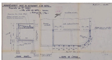
Agrandissement salle de restaurant : coupes, 1966 Repr. Denys Harreau IVR82_20147300892NUCB
