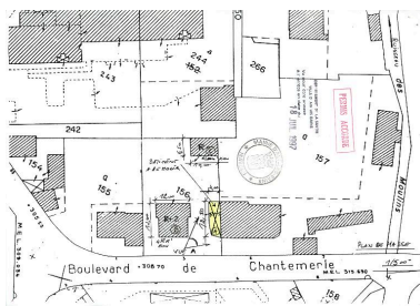
Extension de l'ancienne salle de restaurant : plan masse avant démolition Repr. Denys Harreau IVR82_20137301172NUCB
