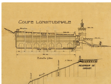
Coupe longitudinale Repro. François Fouger IVR82_20077300891NUCB
