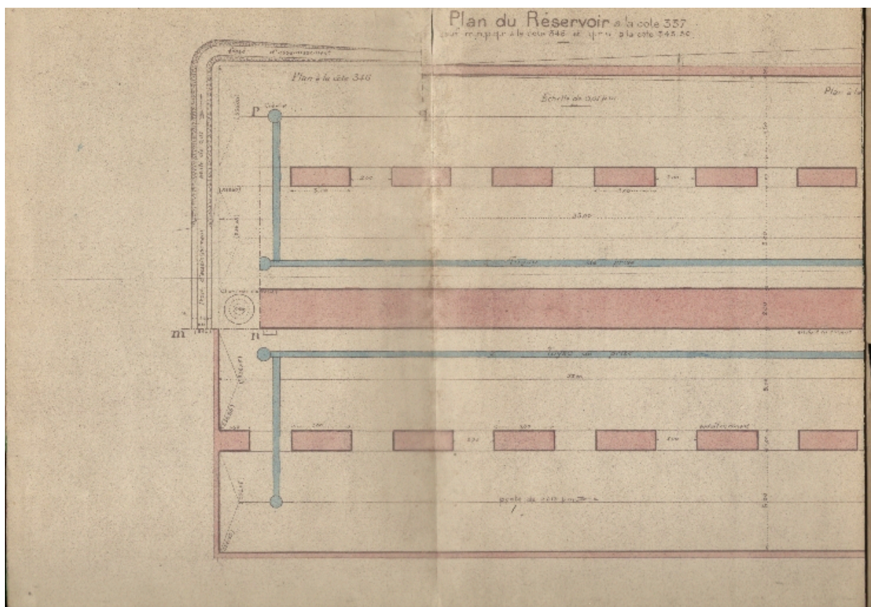
Plan du réservoir, partie gauche
