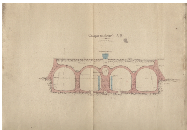
Coupe suivant AB Repro. François Fouger IVR82_20087300794NUCB
