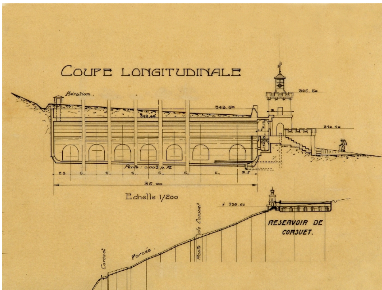
Coupe longitudinale
