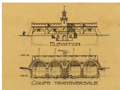
Coupe et élévation Repro. François Fouger IVR82_20077300890NUCB
