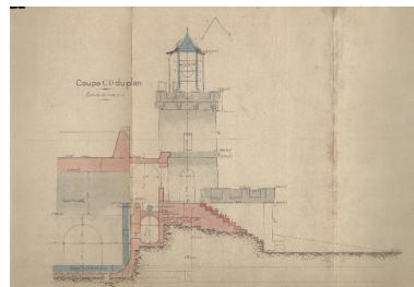
Coupe suivant CD Repro. François Fouger IVR82_20087300795NUCB
