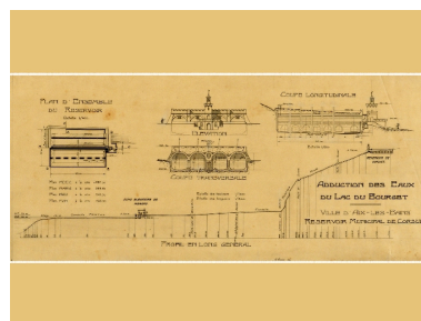
Plans, coupes et élévations Repro. François Fouger IVR82_20077300889NUCB
