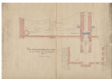
Plan de la chambre d'arrivée Repro. François Fouger IVR82_20087300792NUCB
