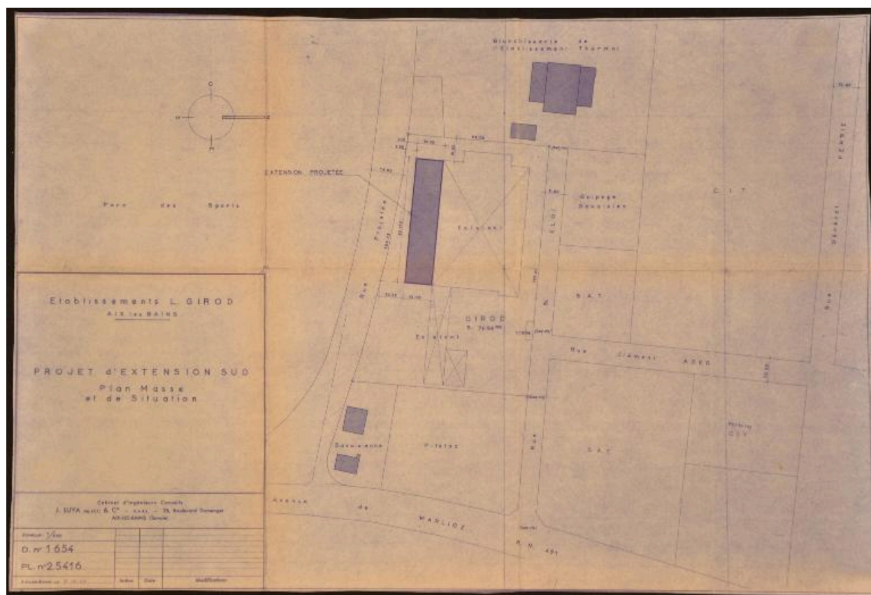
Etablissement L. Girod et blanchisserie. Plan masse, 1963
