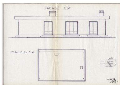
Logement de gardien : façade est Repro. François Fouger IVR82_20127300665NUCB
