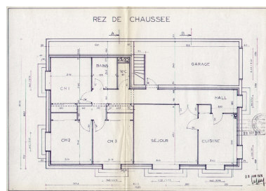
Logement de gardien : rez-de-chaussée Repro. François Fouger IVR82_20127300664NUCB
