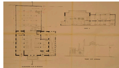
Projet non réalisé. Plan, élévation et coupe du bâtiment existant, 1967 Repro. Denys Harreau IVR82_20137300503NUCB
