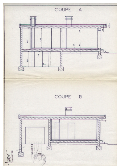
Logement de gardien : coupes Repro. François Fouger IVR82_20127300667NUCB
