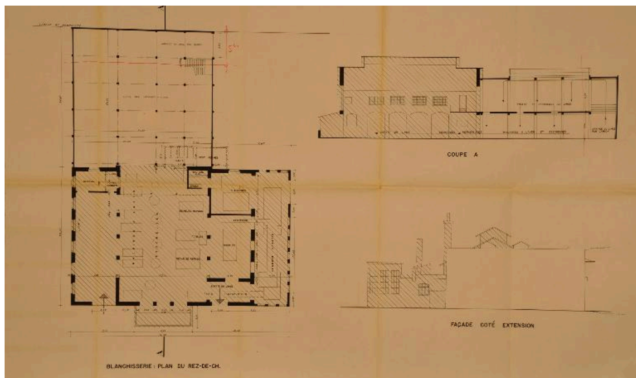
Projet non réalisé. Plan, élévation et coupe du bâtiment existant, 1967
