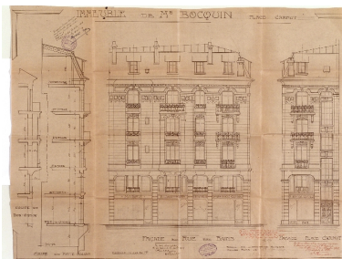
Elévations et coupes Repro. François Fouger IVR82_20057300290NUCB
