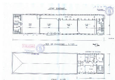
Plans du rez-de-chaussée et de l'étage avant transformation Repro. François Fouger IVR82_20097300441NUCB
