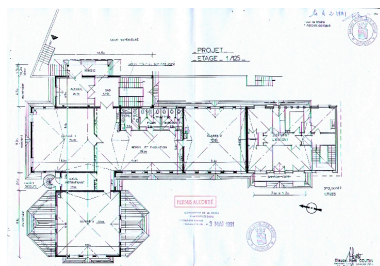
Plan de l'étage, projet Repro. François Fouger IVR82_20097300446NUCB
