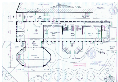
Plan du rez-de-chaussée, projet Repro. François Fouger IVR82_20097300445NUCB
