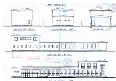
Elévations et coupe avant transformation Repro. François Fouger IVR82_20097300442NUCB
