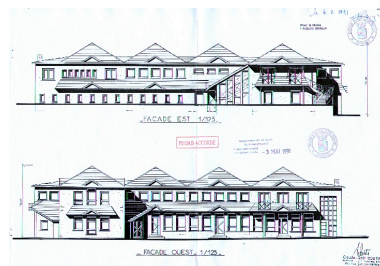
Elévations est et ouest, projet Repro. François Fouger IVR82_20097300447NUCB
